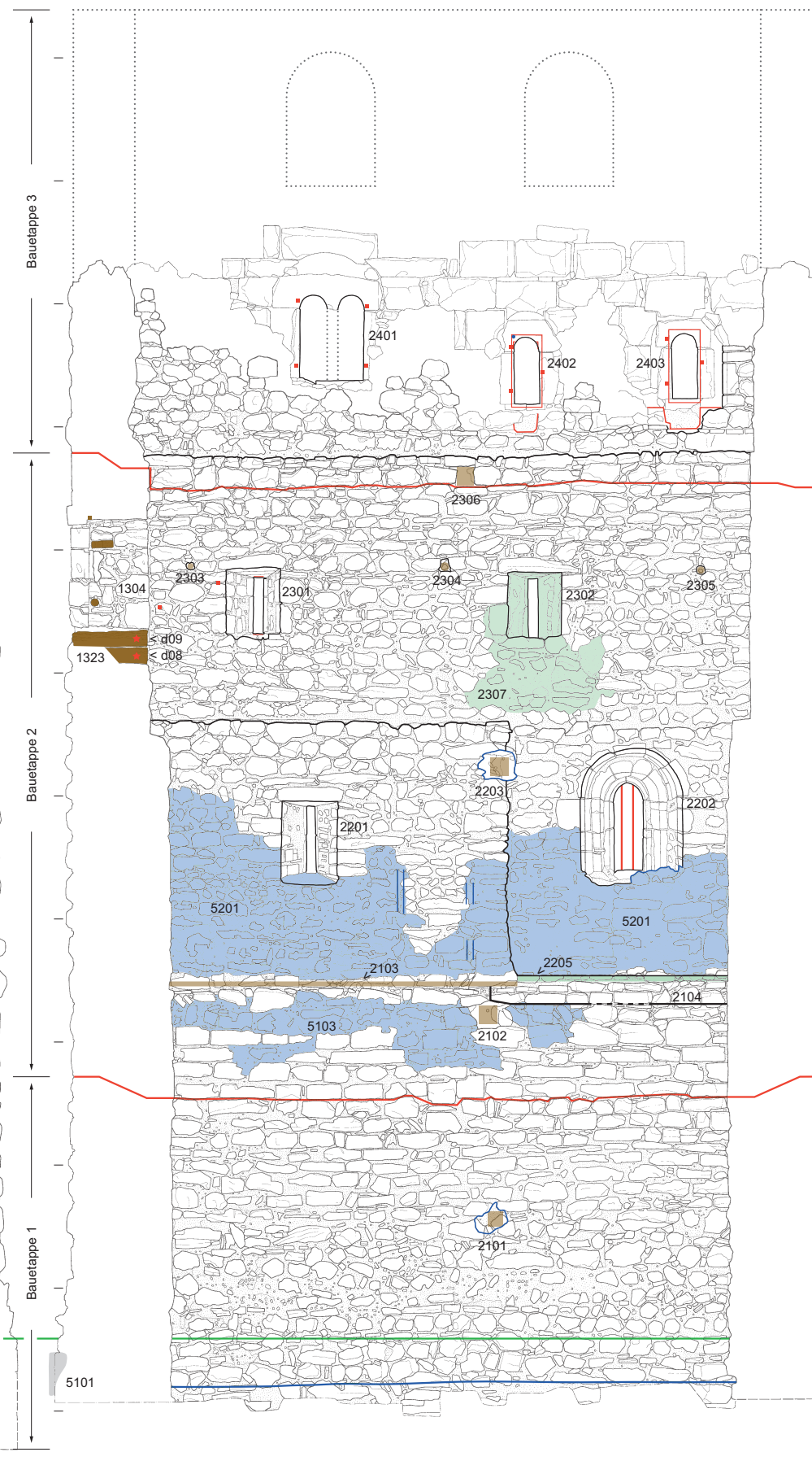
Ansicht Ost
