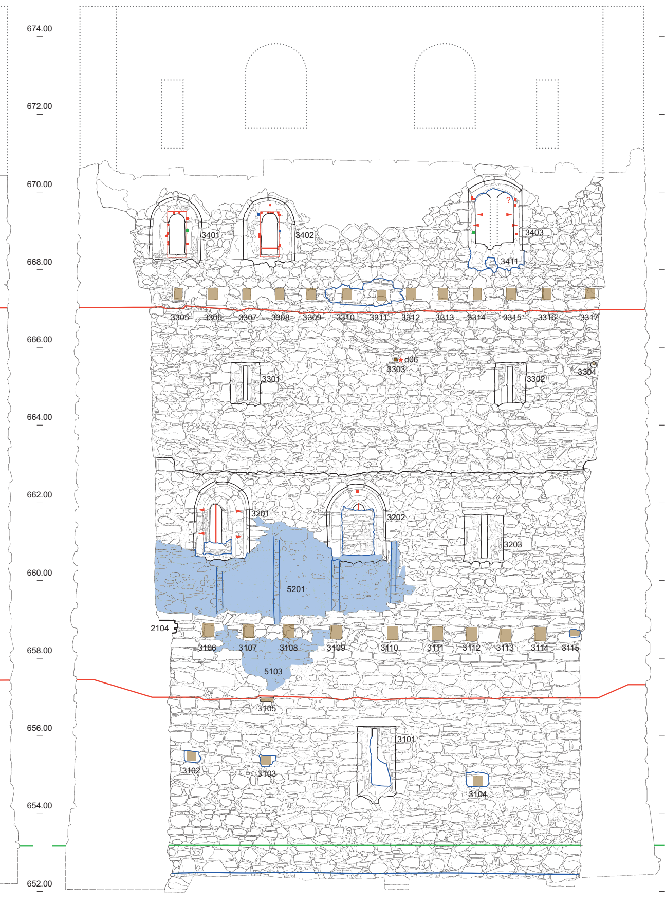
Ansicht Süd
