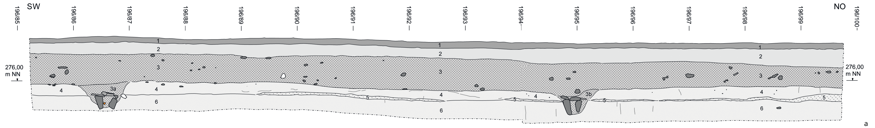
Mendig, »Im Winkel«. Westprofil von Schnitt 1 mit Drainageleitungen. – Sedimente: 1 dunkelbrauner Lehm; 2 grauer Lehm mit einzelnen Rostflecken; 3 dunkelgrauer Lehm mit zahlreichen Steinchen (vor allem Schiefer) und einigen Basaltsteinen; 3a wie 3, aber stellenweise mit lehmigen Lagen, etwas dunkler und grauer als 4 und 6; 3b etwas dunkler als 3, Rostband bildet Grenze zu 4, keine deutliche Grenze zu 3 und zu 6; 4 grauer Lehm mit wenigen Steinchen und einzelnen Rostflecken; 5 etwas mehr Steinchen als 4 und 6, sowie etwas Holzkohle; 6 grauer Lehm mit Rostflecken entlang von Wurzelbahnen. – (Grafik S. Wenzel). – M. 1:40.
