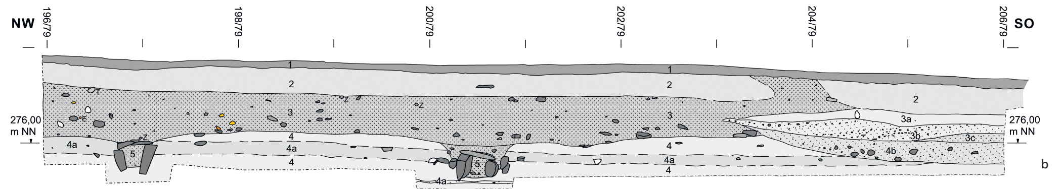
Mendig, »Im Winkel«. Nordprofil von Schnitt 2 mit Drainageleitungen und spätmittelalterlichen bis neuzeitlichen Bachsedimenten; am Südost-Ende vermutlich durch Baumwurf überprägt. – Sedimente: 1 dunkelbrauner Lehm; 2, 3a grauer Lehm mit einzelnen Rostflecken; 3 dunkelgrauer Lehm mit zahlreichen Steinchen (vor allem Schiefer) und einigen Basaltsteinen; 3b grauer Grobsand und Kies in wechselnden Anteilen, an der Basis teils rostfarben; 3c grauer Lehm mit einzelnen Rostflecken und einigen Steinchen, keine deutliche Grenze zu 4; 4 grauer Lehm mit einzelnen Steinchen und einigen Rostflecken; 4a wie 4, aber etwas mehr Steinchen und »grauer«; 4b wie 4, aber mit Basaltbrocken und etwas mehr Steinchen; 5 wie 3, aber nach unten hin Rostbändchen. – (Grafik S. Wenzel). – M. 1:40.
