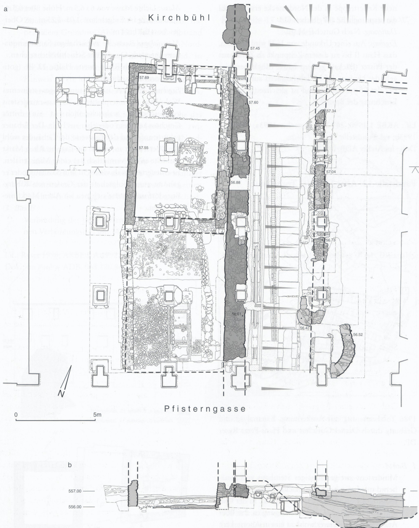
Abb. 182: Fundstelle 11 Marktaube. a Grundriss, dunkler Raster: Stadtmauer (Phase 2); mittlerer Raster: Angebautes gründungszeitliches Haus II (Phase 3); heller Raster: Füllung des Grabens (Phase 5) und Bau der Brotschal (Phase 6); b Profil E-W.
