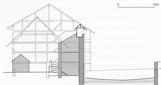
Abb. 179: Fundstelle 8 Metzgergasse 1/3. Rekonstruktion der ursprünglichen Bebauung nach Verf. In Grau hinterlegt der Forschungsstand 1985 (Kdm Bern Land I).
