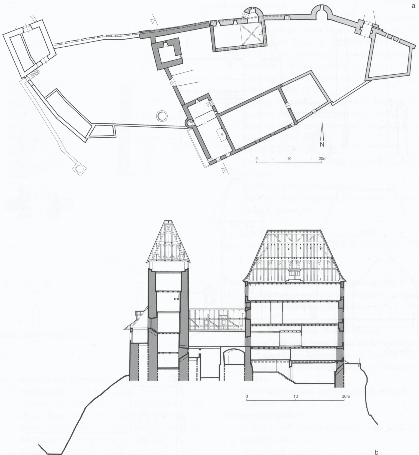
Abb. 176: Fundstelle 5 Schloss. Rekonstruierter Grundriss und Schnitt. Dunkler Raster: Anlage II um 1200, heller Raster: Anlage IIa, mittleres 13. Jahrhundert.
