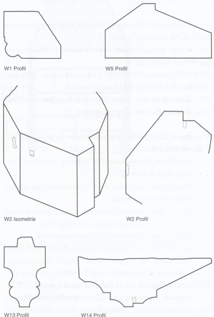
Abb. 175: Fundstelle 4 Stadtkirche. Architekturfragmente von Bau I und von der gotischen Erneuerung des Chors (W 13 und W 14).
