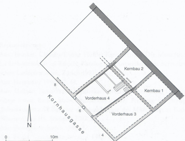
Abb. 192: Fundstelle 29 Kornhausgasse 6. Schematischer Grundriss im ersten Obergeschoss.
