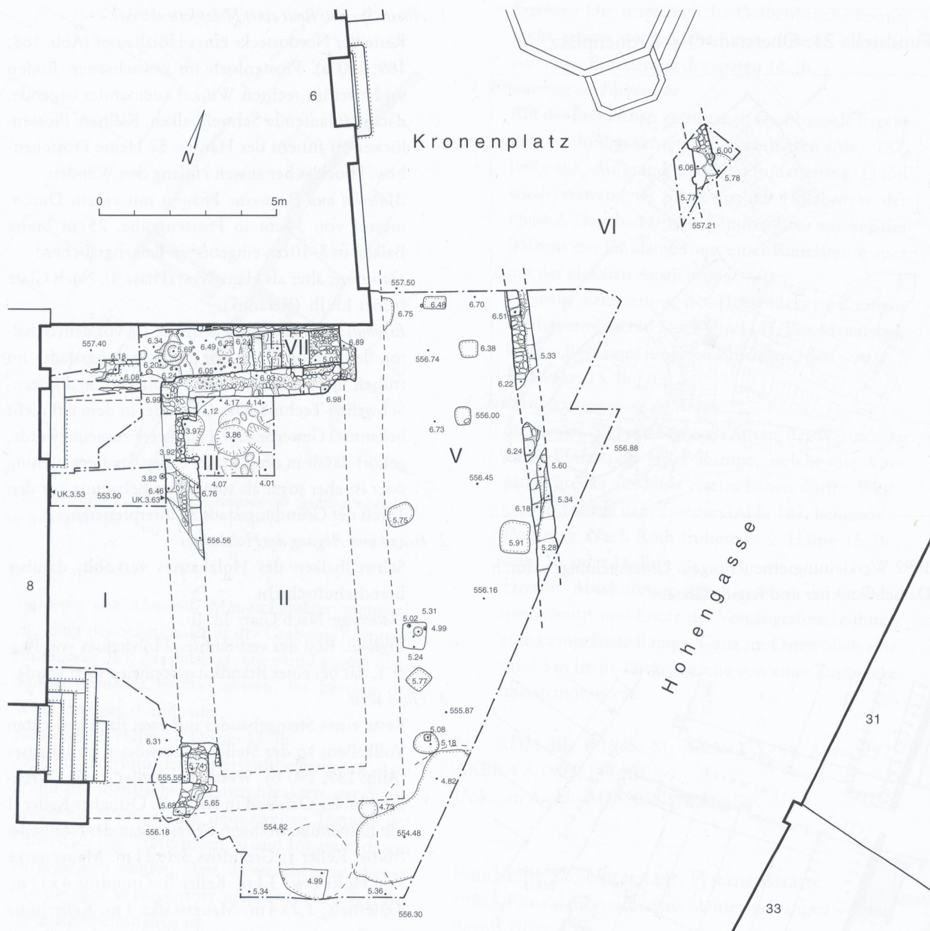
Abb. 189: Fundstelle 23 Kronenplatz. Steingerechter Grundriss.
