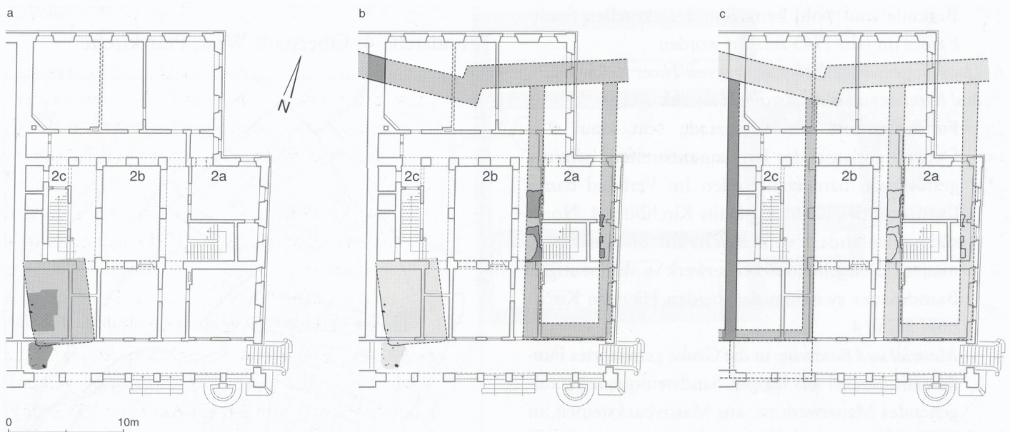
Abb. 173: Fundstelle 2 Stadthaus. a Phasen 1 und 2; b Phasen 3-5; c Phase 6. Dunkler Raster: Befund; heller Raster: Ergänzung.
