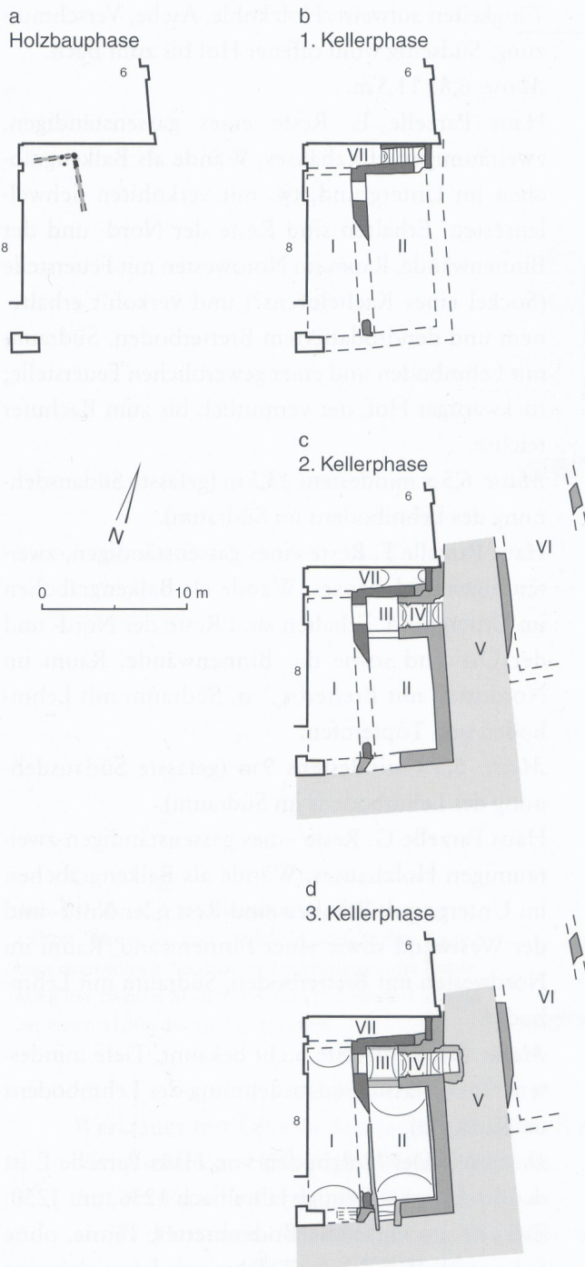
Abb. 190: Fundstelle 23 Kronenplatz. Bauphasenplan.
