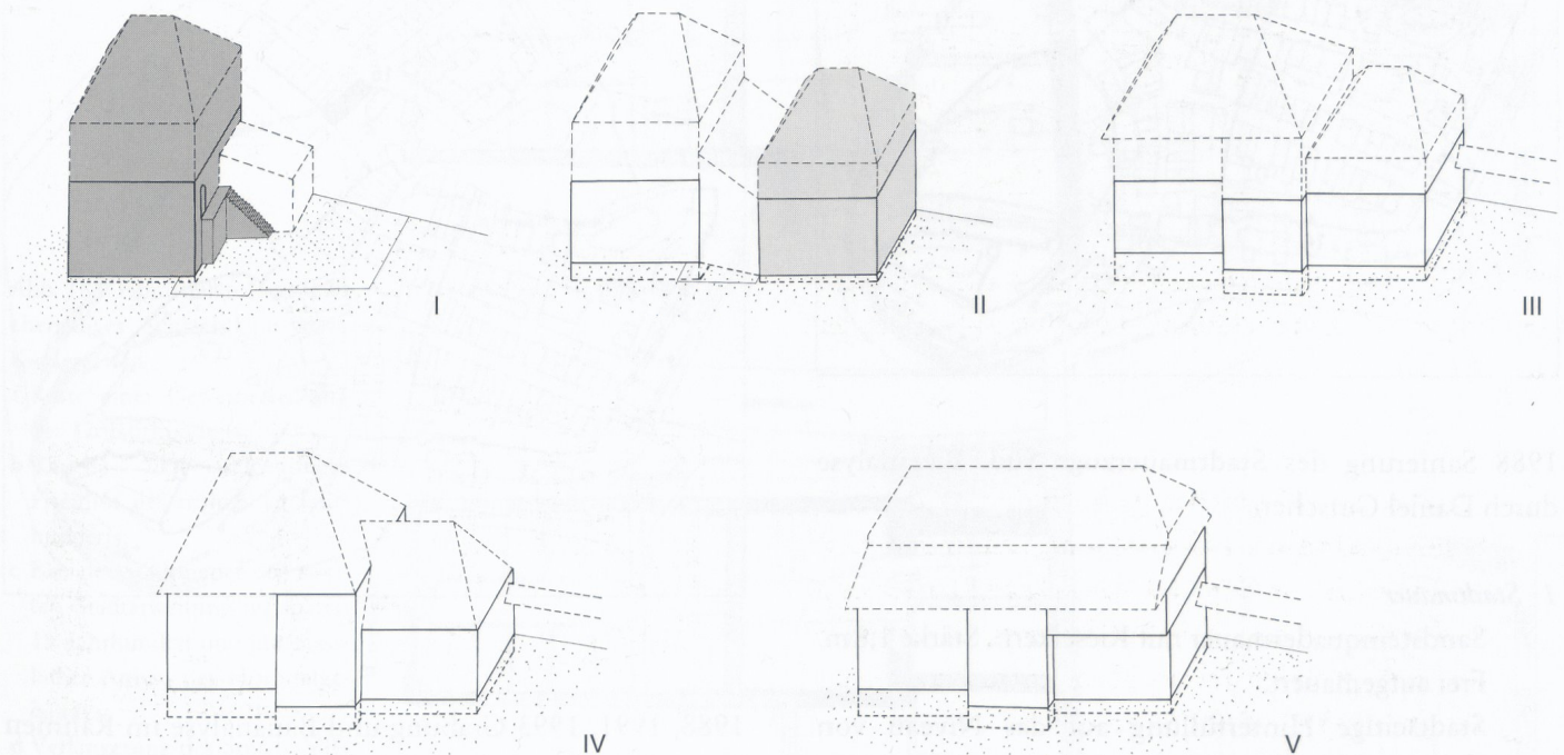
Abb. 183: Fundstelle 12 Trüberhaus. Nordfassade, Grundriss und Rekonstruktion der Gebäudeentwicklung.
