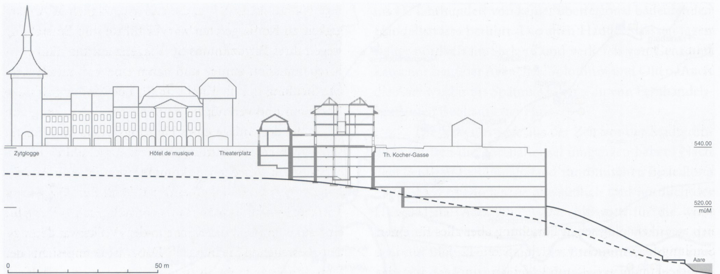
Abb. 102: Bern. Längsschnitt durch den südlichen Teil des natürlichen Quergrabens auf der Linie Kornhausplatz-Theaterplatz-Casinoplatz. Die Häuserzeile Ost ist in Ansicht, die alte Hauptwache und der Komplex Winterthurhaus/Bellevue-Garage (Casinoparking) im Schnitt gezeichnet. Der Graben ist mindestens 10m tief; gegen Süden nimmt er rasch an Tiefe zu und zieht bis an das Aareufer hinunter.
