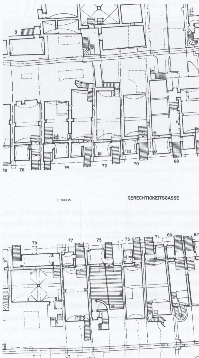
Abb. 122: Bern, «Kellerplan der Berner Altstadt». Grundriss der Bereiche Gründungsstadt, Innere und Äussere Neuenstadt auf dem Kellergeschossniveau, Zustand 1980, 1:500, Ausschnitt. Baugeschichtliche Aussagen fehlen auf dem Plan.
