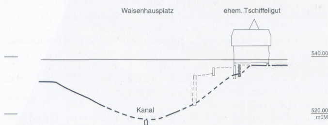
Abb. 104: Bern. Querschnitt durch den nördlichen Teil des Grabens auf der Linie Bundesplatz-Bärenplatz-Waisenhausplatz. Gerastert die mittelalterliche Grabenmauer West und das zugehörige Aussenniveau. In dünnen Linien: das spätmittelalterlich-frühneuzeitliche Tschiffelgut mit zugehöriger Gartenterrassierung am Grabenhang. Nach Martin Portmann und Verf.
