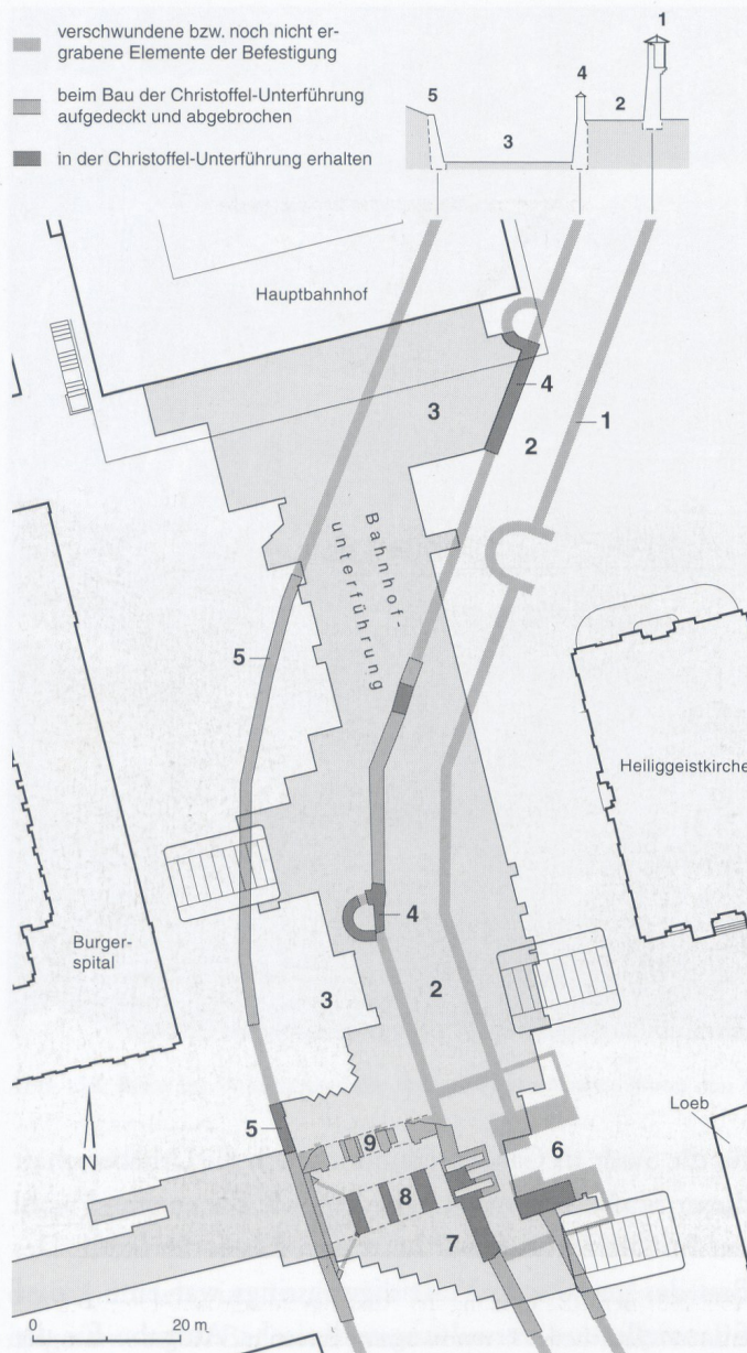
Abb. 160: Bern. Befestigung der Äusseren Neuenstadt. 1 Stadtmauer mit Flankenturm; 2 Rondelweg; 3 Graben; 4 innere Grabenmauer mit Flankenturm; 5 äussere Grabenmauer; 6 Torturm («Christoffel»); 7 Vorwerk; 8 Grabenbrücke; 9 Aquädukt für den Stadtbach.
