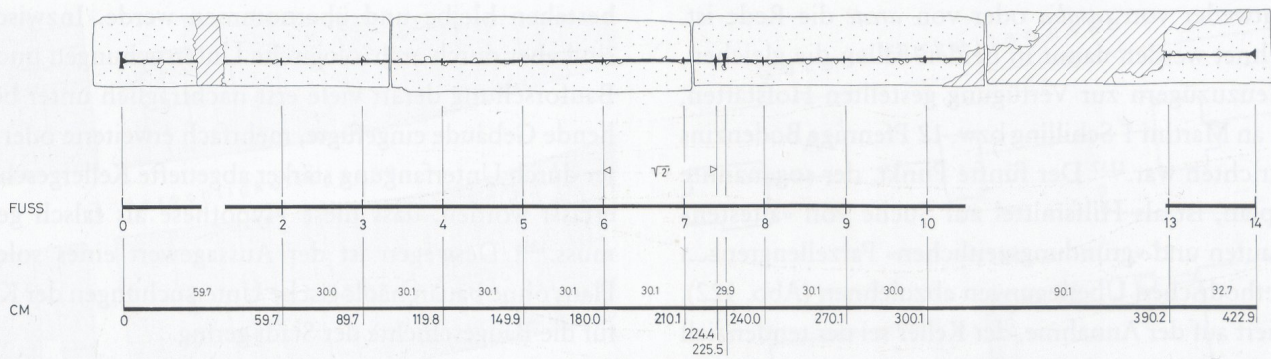
Abb. 120: Bern. Innere Neuenstadt, Dominikanerkloster. An der Lettnerrückwand in der Kirche wurde bauzeitlich eine Messstrecke für die Bauleute eingehauen. Das dort zugrunde liegende mutmassliche Fussmass betrug 30 cm. Damit wurde wahrscheinlich das für den Bau der Kirche verbindliche Fussmass definiert. Ob dieses Mass aber etwas mit dem damals in Bern gebräuchlichen zu tun hat, ist völlig ungewiss. Es entspricht jedenfalls nicht dem im 17. Jh. in Bern gebräuchlichen Fussmass (29,3 cm nach Tuor 1977), welches Grundlage der Hoferschen und Strahmschen Hypothesen ist.
