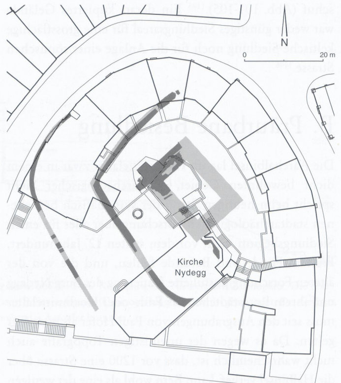
Abb. 106: Bern, Nydegghöfli. Grabungsgrundriss der Burg Nydegg. Mit den Grundrissen der heutigen, 1951–1962 entstandenen Wohnbebauung um den Burghügel und der Nydeggkirche.
