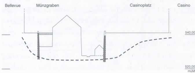
Abb. 103: Bern. Querschnitt durch den südlichen Teil des Grabens auf der Linie Kornhausplatz-Theaterplatz-Casinoplatz auf der Höhe Kochergasse im Jahr 1935, unmittelbar vor dem Bau der Bellevue-Garage. Gestrichelt die Hangkanten des Grabens, gerastert die mittelalterlichen Grabenmauern. Im Graben in schematischer Darstellung die alte Bebauung mit Gerberhäusern und Stadtbachableitung.
