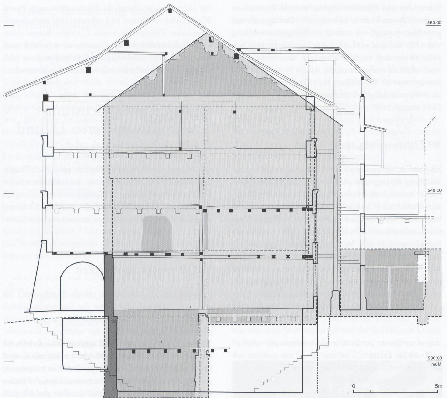
Abb. 154: Bern, Gerechtigkeitsgasse 71. Schnitt durch das Gebäude mit Ansicht der ostseitigen Brandmauer und der Ostmauer des rückwärtigen Hofes von 1265d nach Verf. Dunkler Raster: Schnittfläche, Befund; mittlerer Raster: Befunde; heller Raster: Rekonstruktion.
