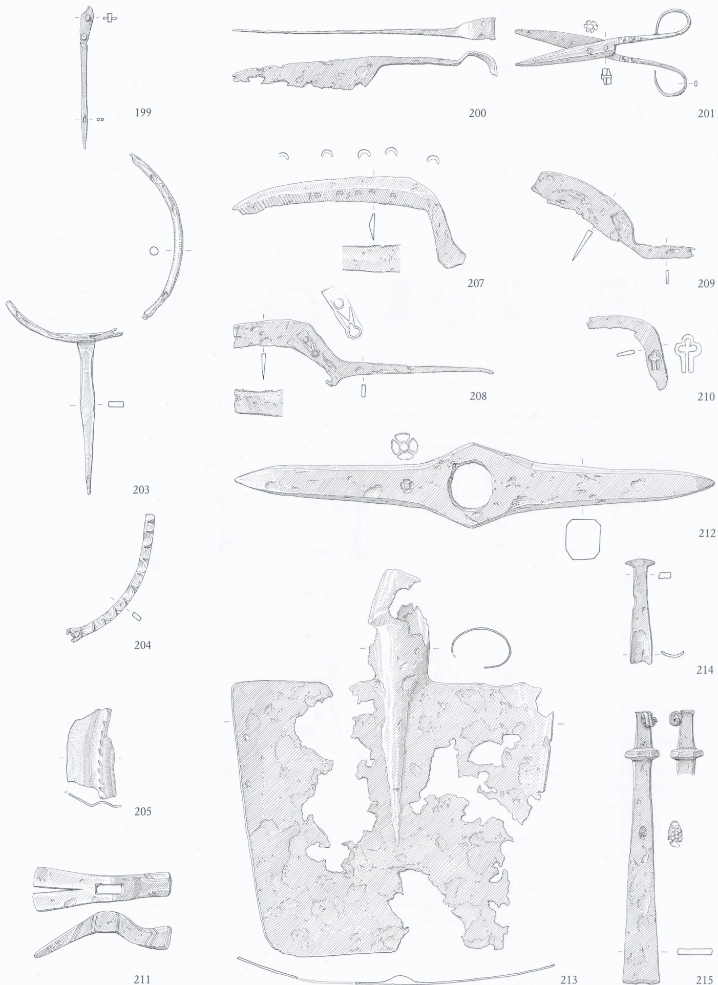
Tafel 19 199–206 Essbesteck, Scheren und Küchengeräte (202 siehe Abb. 151, 206 siehe Abb. 152), 207–215 Werkzeuge und landwirtschaftliche Geräte. 205 Mst. 1:2, übrige Mst. 1:3, Schlagmarken Mst. 2:3.
