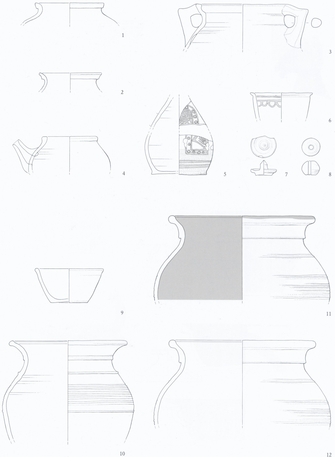
Tafel 1 1-7, 9-12 Geschirrkernik, 8 Spinnwirtel. Mst. 1:3.
