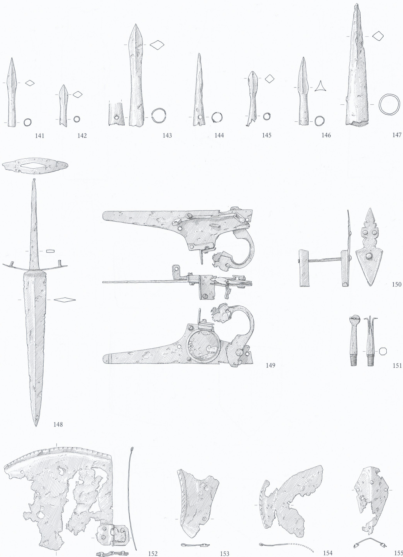
Tafel 16 141–155 Waffen und Rüstungsteile. Mst. 1:3.
