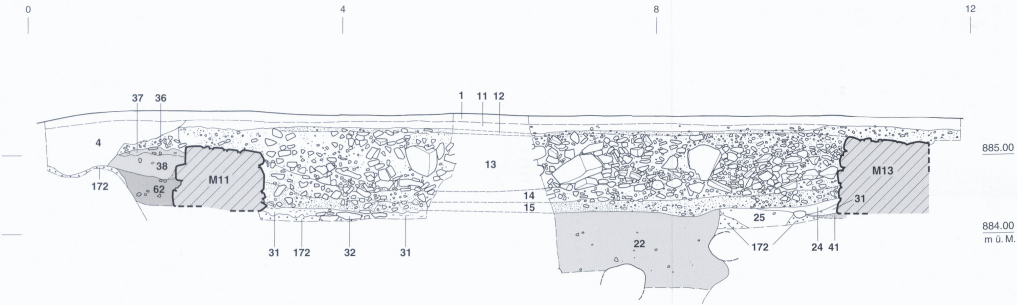
Profil P6, M. 1:50.
