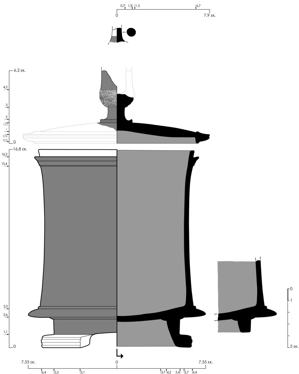
Πίν. 10. Η πυξίδα, οψοτομή με μετρήσεις.
