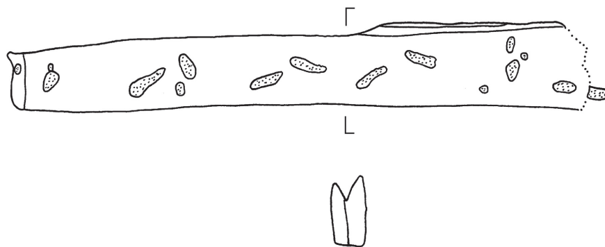
Abb. 67b. – Wrack 4. Spanten A 8* bis A 11*. – M. 1:10.
