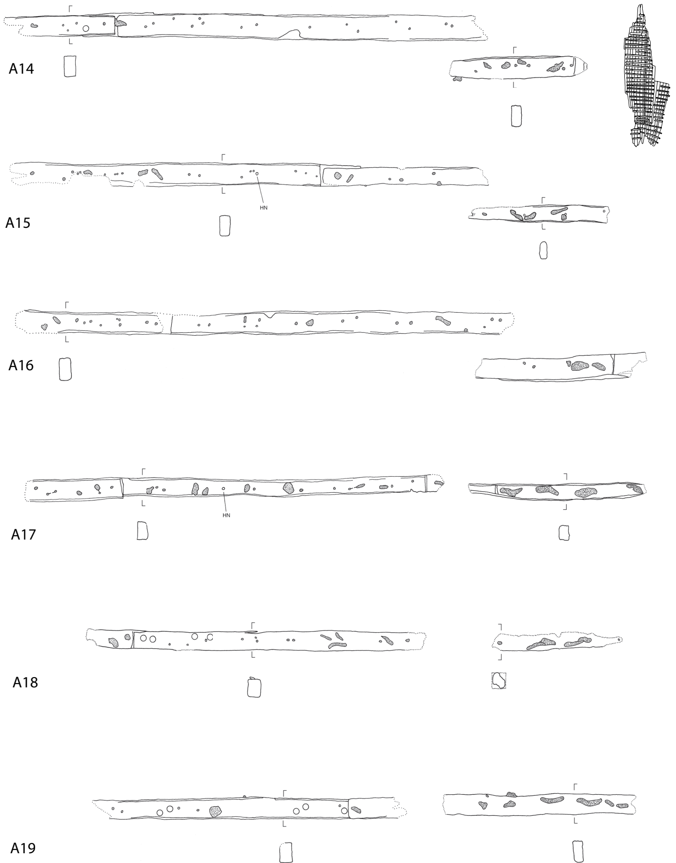
Abb. 62b. – Wrack 3. Spanten A 14 bis A 19. – M. 1:20.
