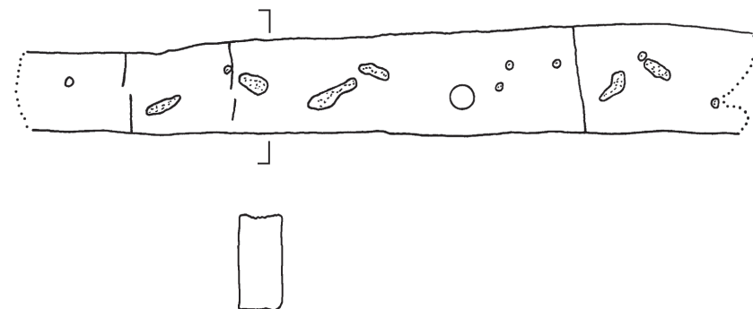
Abb. 68b. – Wrack 4. Spanten A 8* bis A 11*. – M. 1:10.
