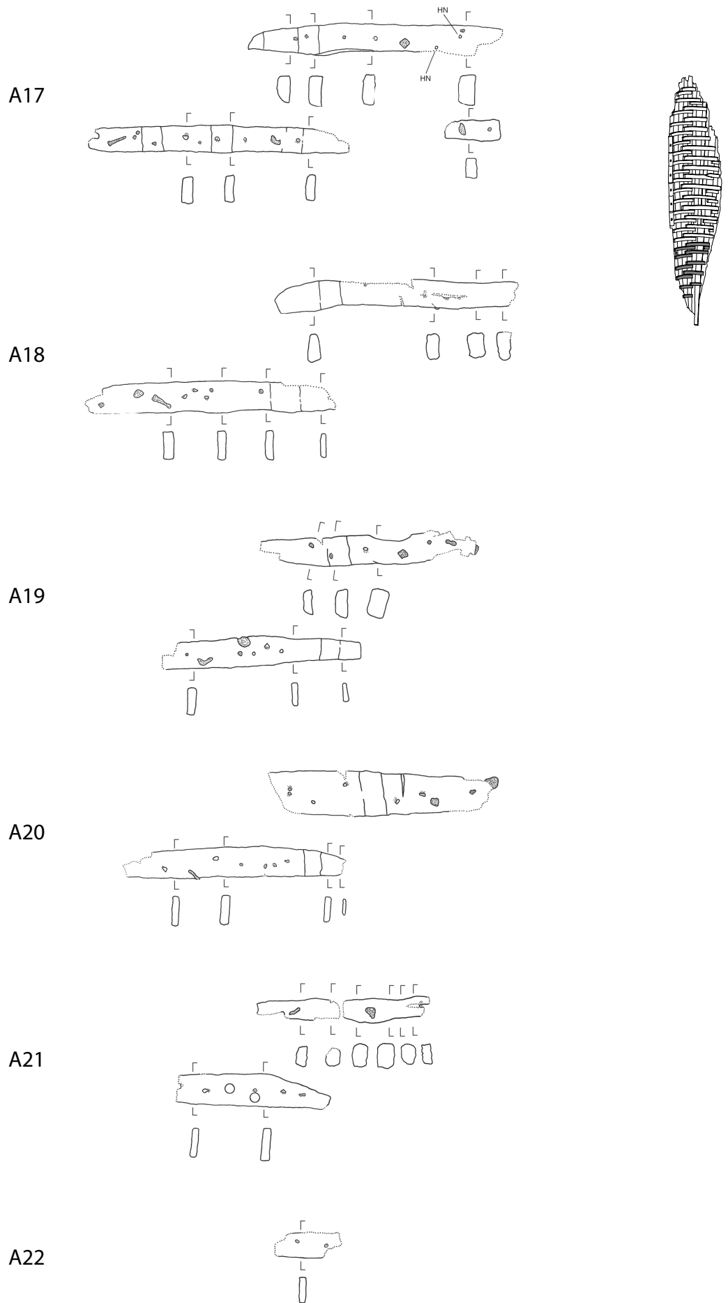
Abb. 53b. – Wrack 1. Spanten A 17* bis A 12*. – M. 1:20.
