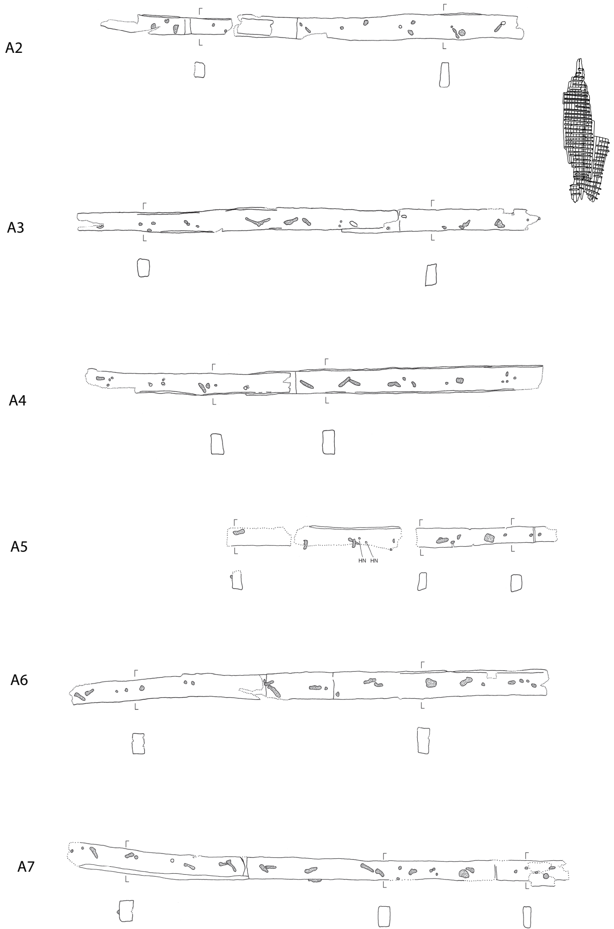
Abb. 60b. – Wrack 3. Spanten A 2 bis A 7. – M. 1:20.
