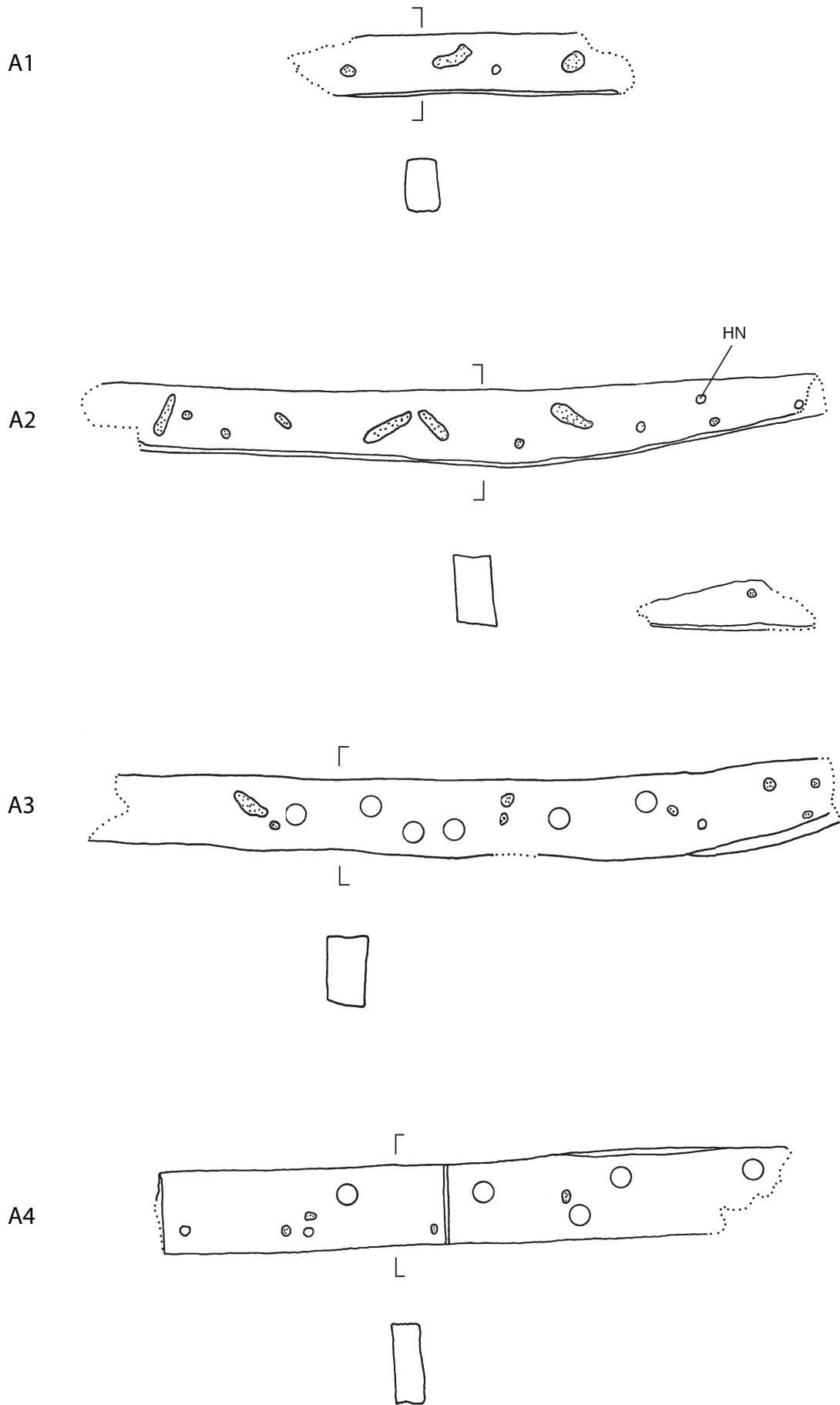
Abb. 65b. – Wrack 4. Spanten A 1* bis A 4*. – M. 1:10.
