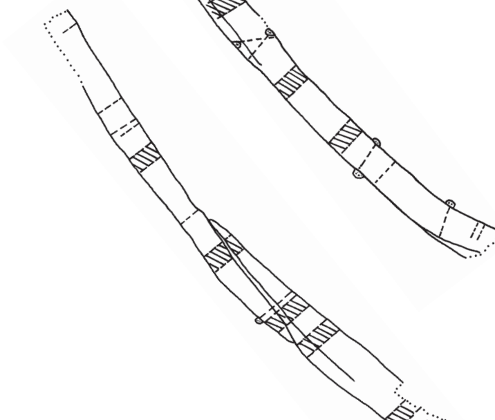
Abb. 65a. – Wrack 4. Spanten A 1* bis A 4*. – M. 1:10.
