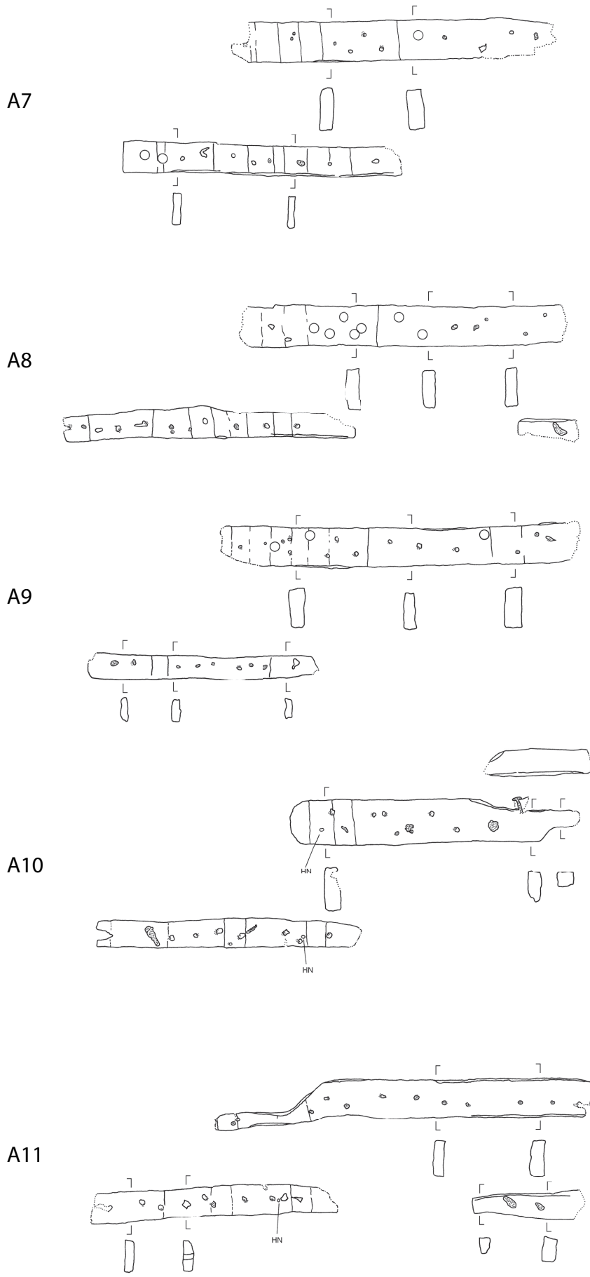
Abb. 51b. – Wrack 1. Spanten A 7* bis A 11*. – M. 1:20.
