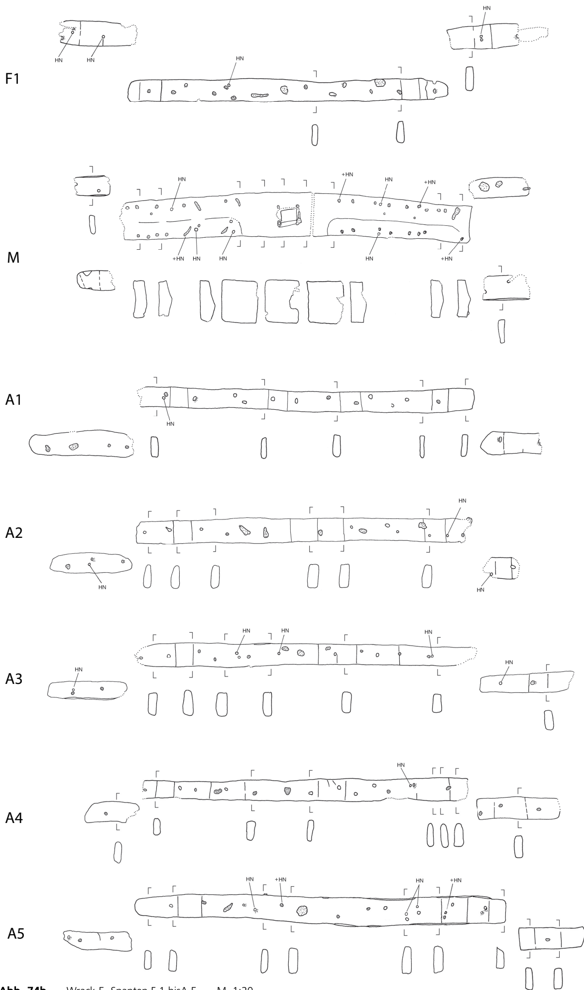
Abb. 74b. – Wrack 5. Spanten F 1 bis A 5. – M. 1:20.
