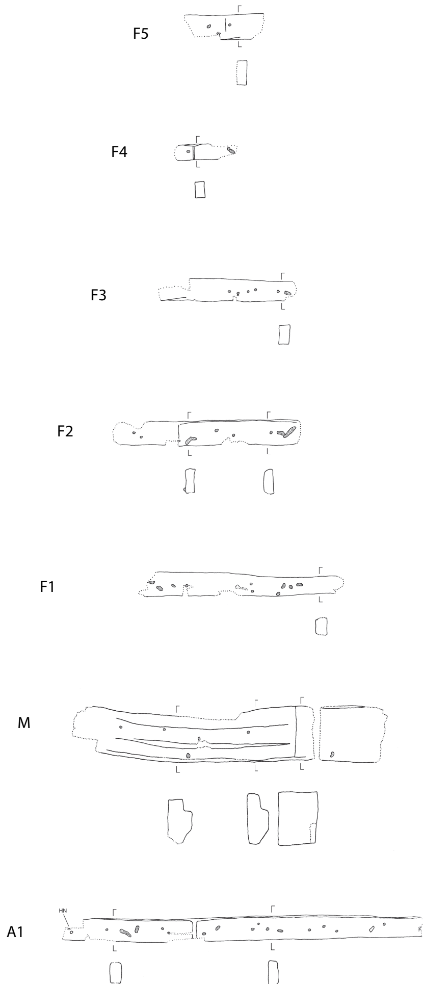
Abb. 59b. – Wrack 3. Spanten F 5 bis A 1. – M. 1:20.
