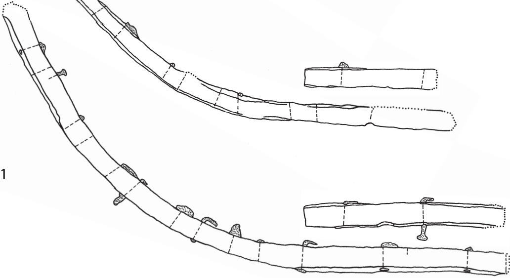
Abb. 55a. – Wrack 2. Spanten A 7* bis A 11*. – M. 1:10.
