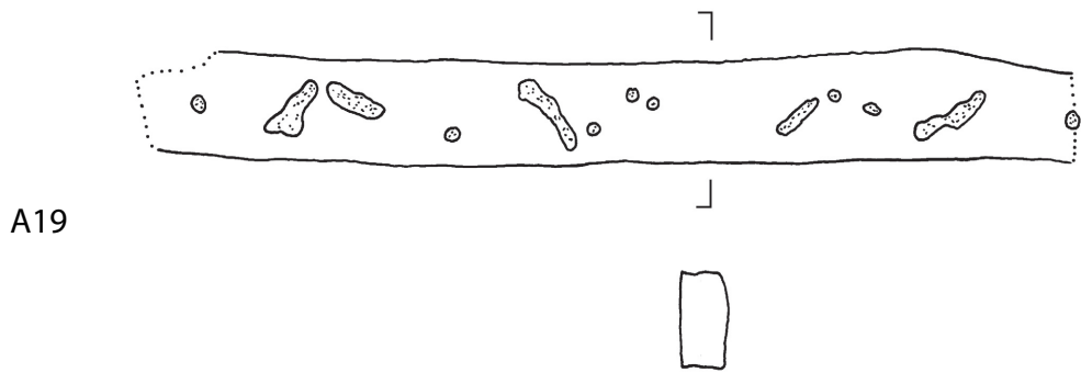
Abb. 69b. – Wrack 4. Spanten A 16* bis A 19*. – M. 1:10.
