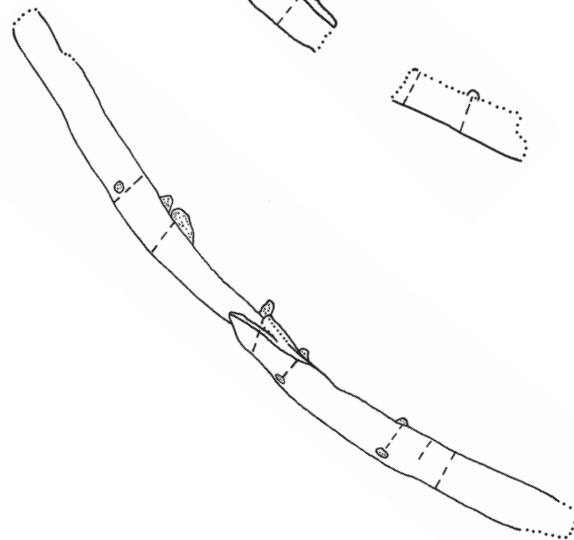
Abb. 54a. – Wrack 2. Spanten A 2* bis A 6*. – M. 1:10.
