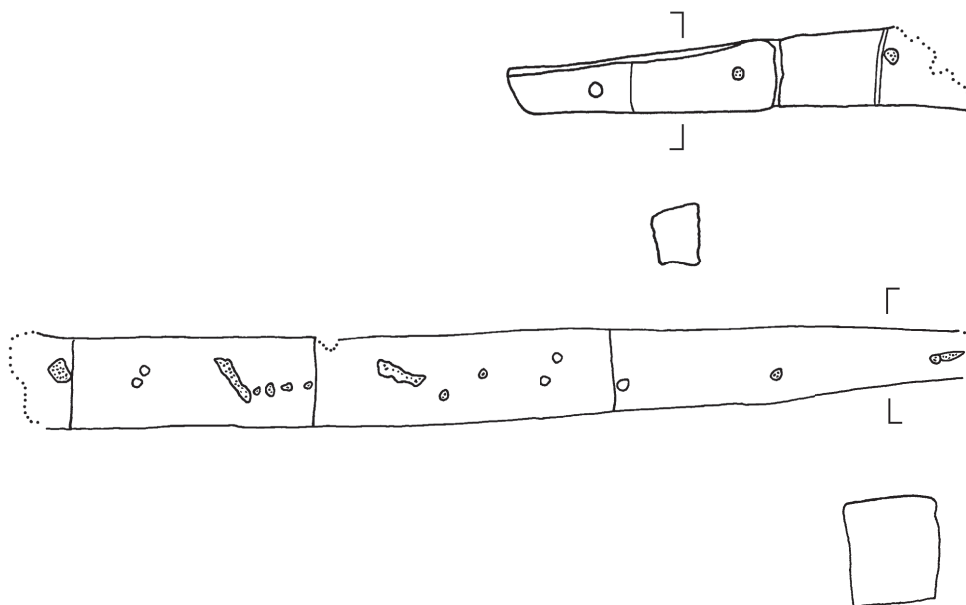
Abb. 66b. – Wrack 4. Spanten A 5* bis A 7*. – M. 1:10.
