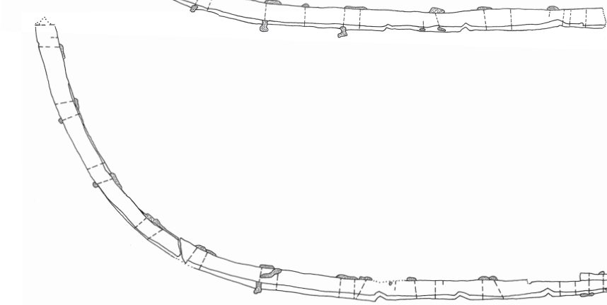
Abb. 60a. – Wrack 3. Spanten A 2 bis A 7. – M. 1:20.
