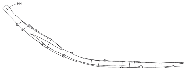
Abb. 59a. – Wrack 3. Spanten F 5 bis A 1. – M. 1:20.
