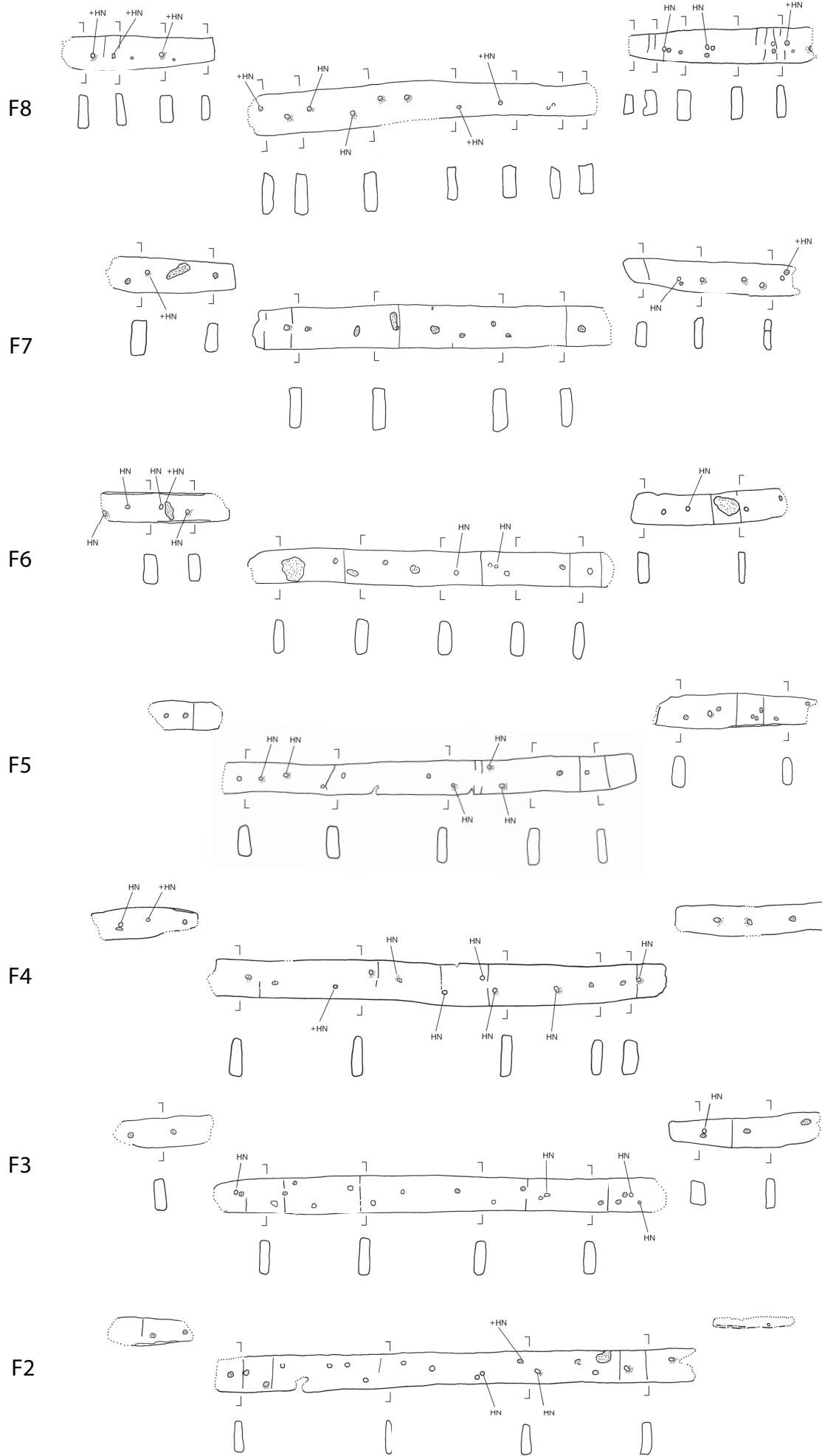
Abb. 73b. – Wrack 5. Spanten F 8 bis F 2. – M. 1:20.
