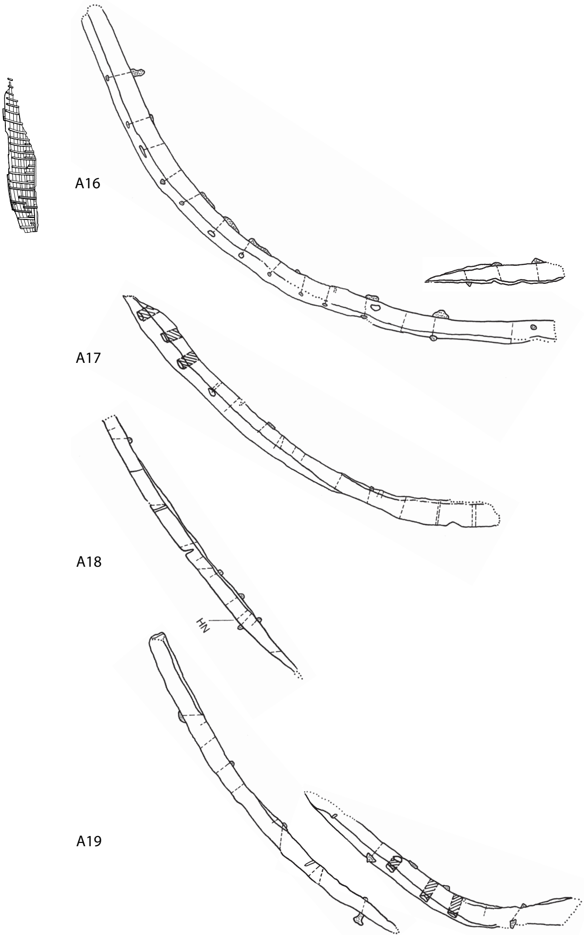
Abb. 57a. – Wrack 2. Spanten A 16* bis A 19*. – M. 1:10.
