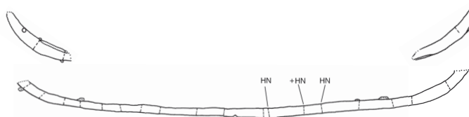
Abb. 73a. – Wrack 5. Spanten F 8 bis F 2. – M. 1:20.
