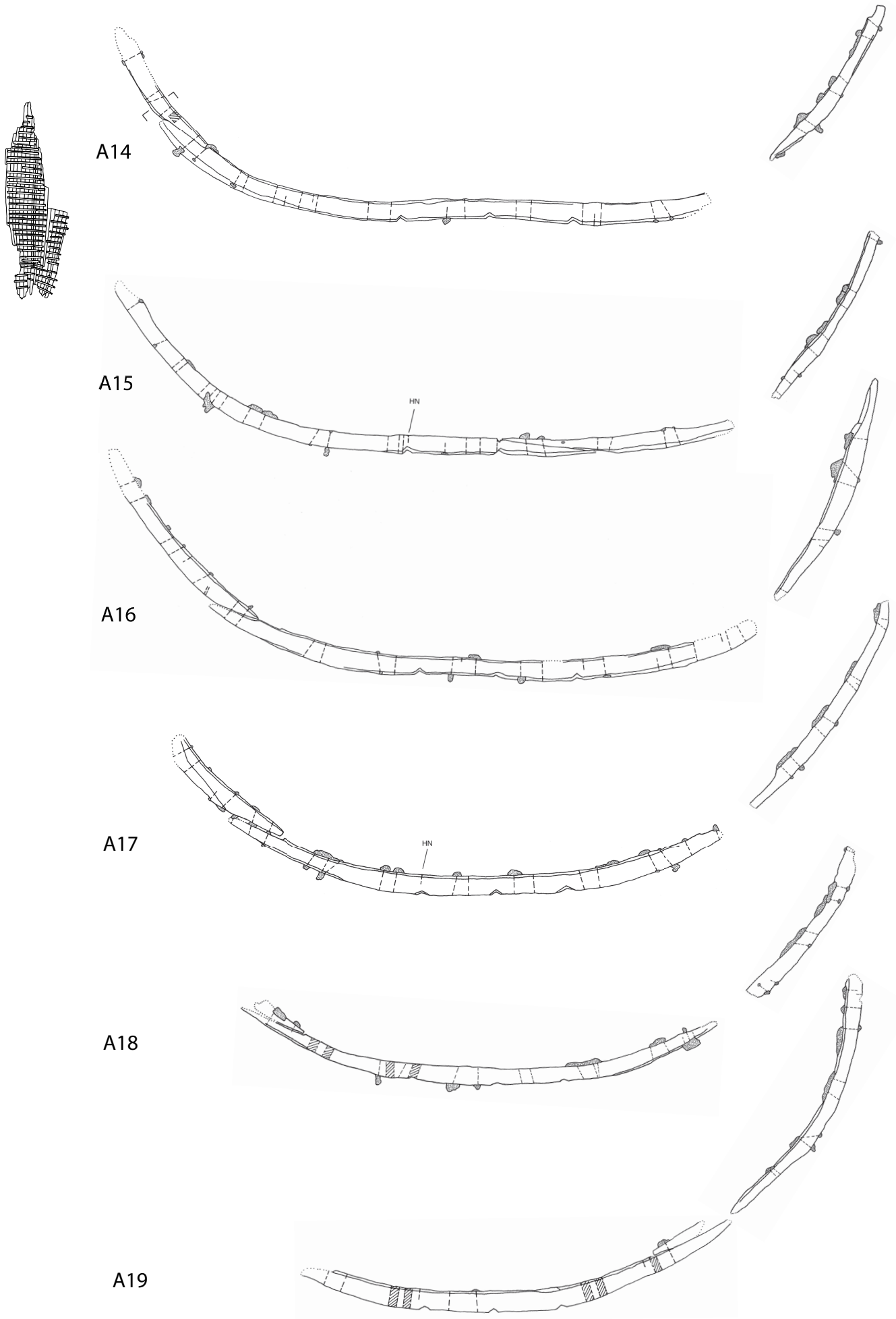
Abb. 62a. – Wrack 3. Spanten A 14 bis A 19. – M. 1:20.
