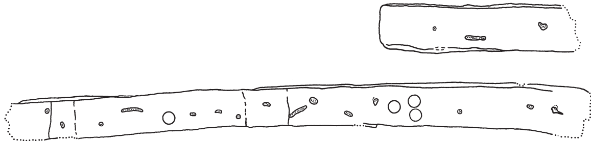
Abb. 56b. – Wrack 2. Spanten A 12* bis A 15*. – M. 1:10.
