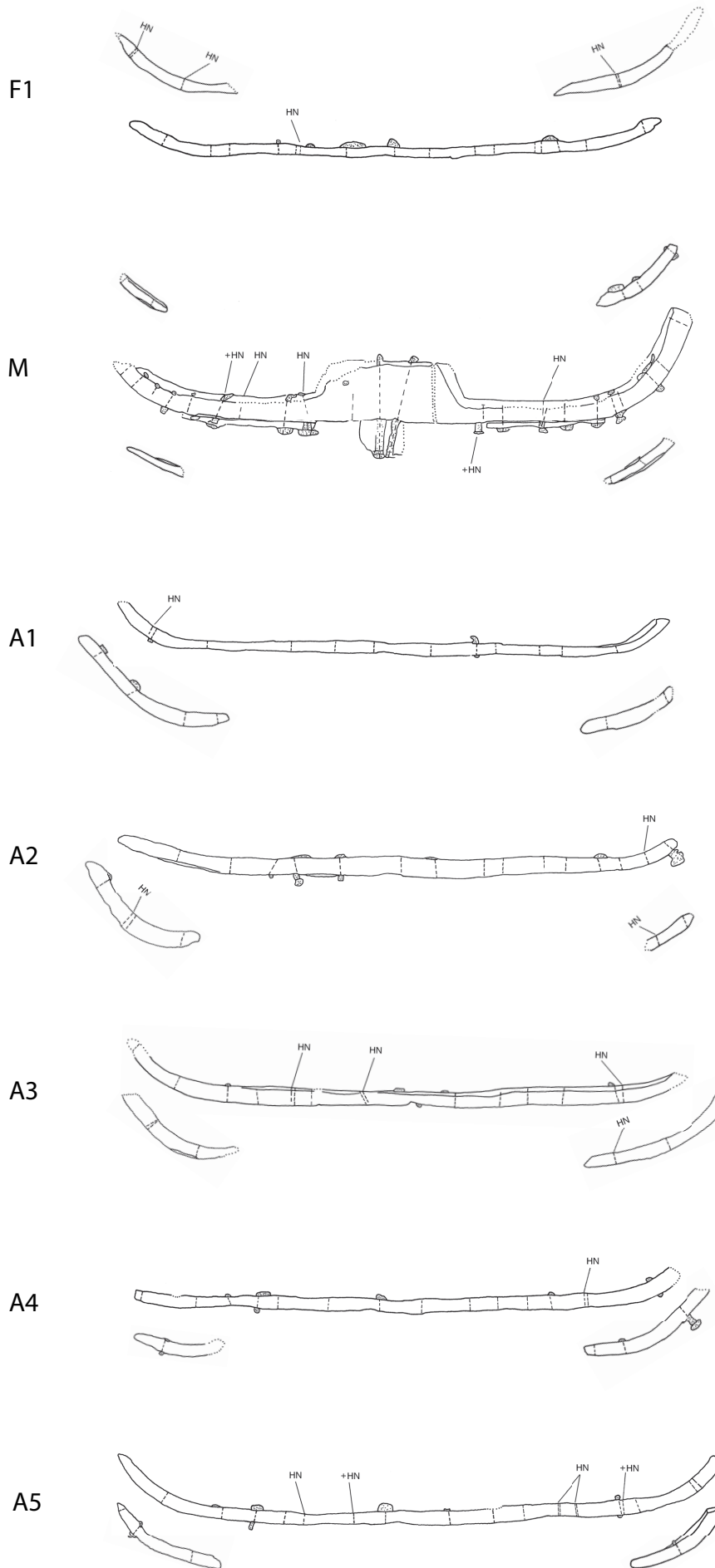
Abb. 74a. – Wrack 5. Spanten F 1 bis A 5. – M. 1:20.
