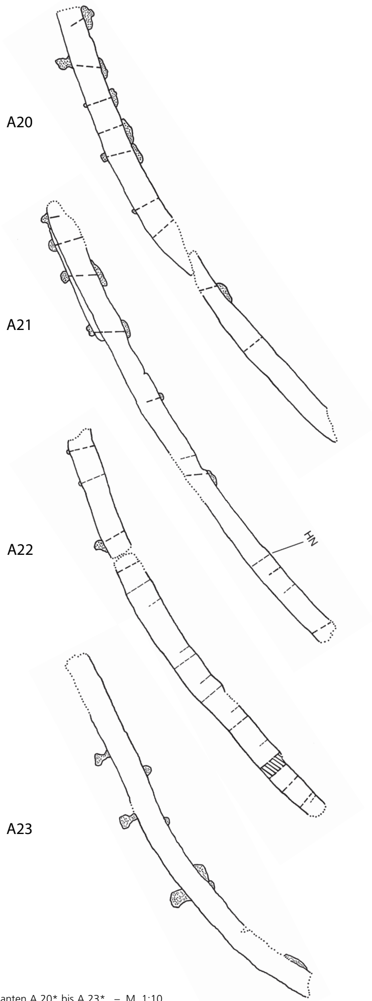
Abb. 70a. – Wrack 4. Spanten A 20* bis A 23*. – M. 1:10.
