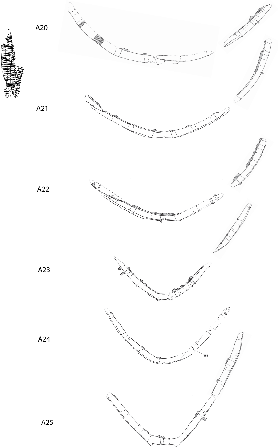
Abb. 63a. – Wrack 3. Spanten A 20 bis A 25. – M. 1:20.
