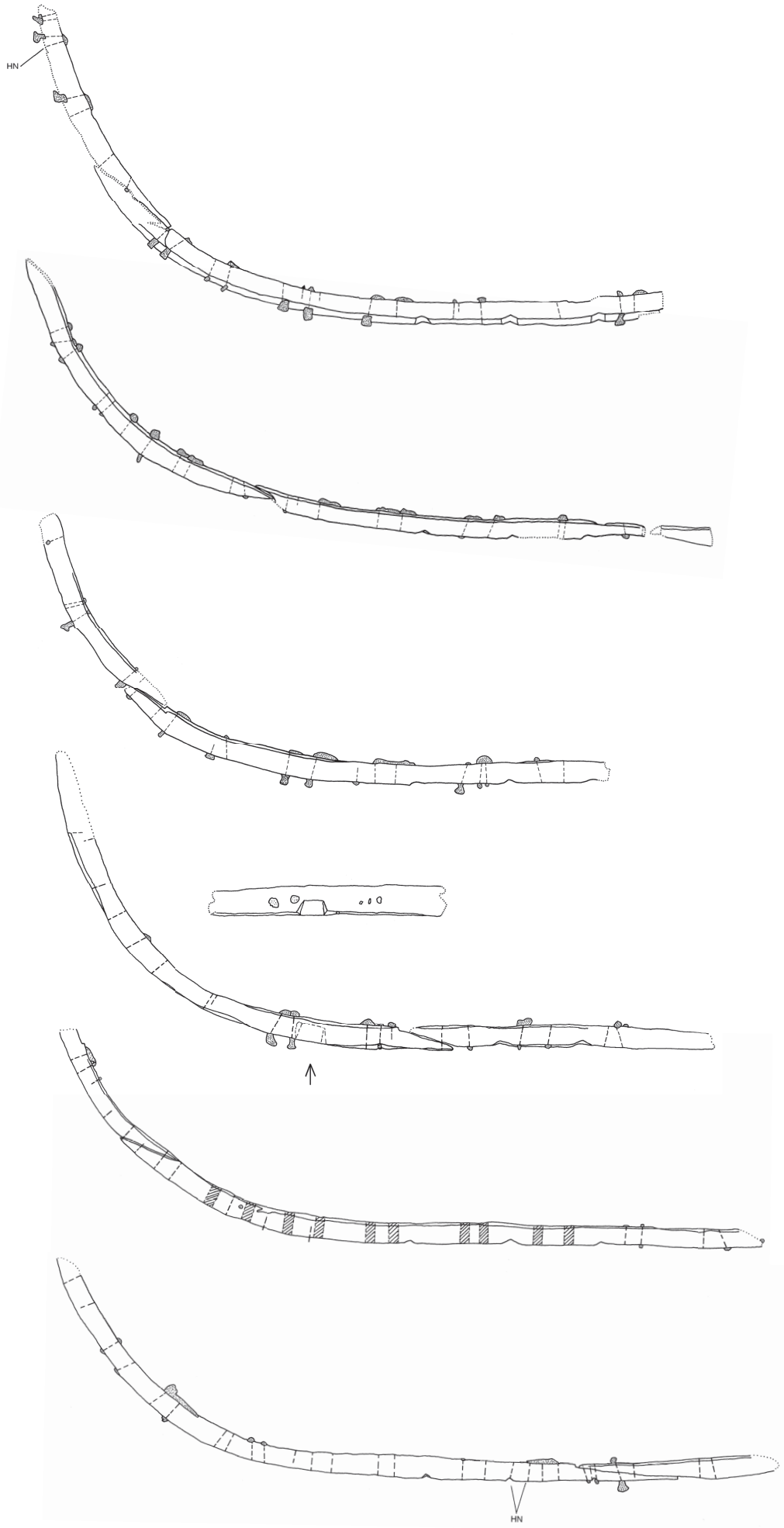
Abb. 61a. – Wrack 3. Spanten A 8 bis A 13. – M. 1:20.
