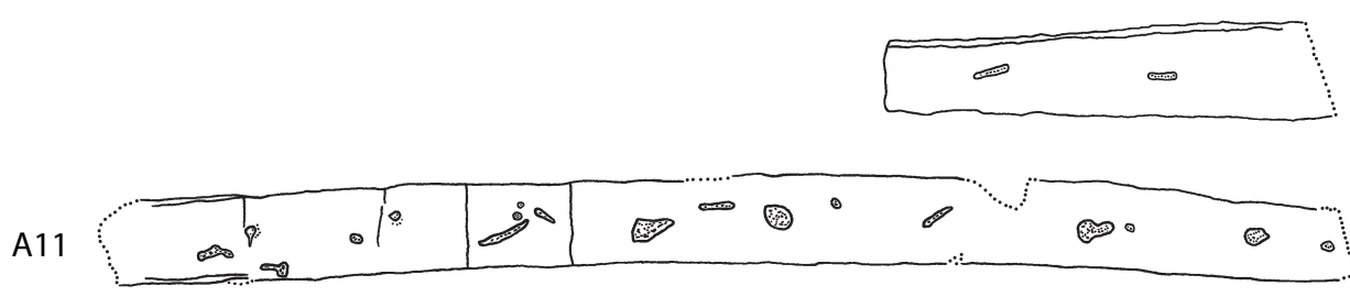
Abb. 55b. – Wrack 2. Spanten A 7* bis A 11*. – M. 1:10.
