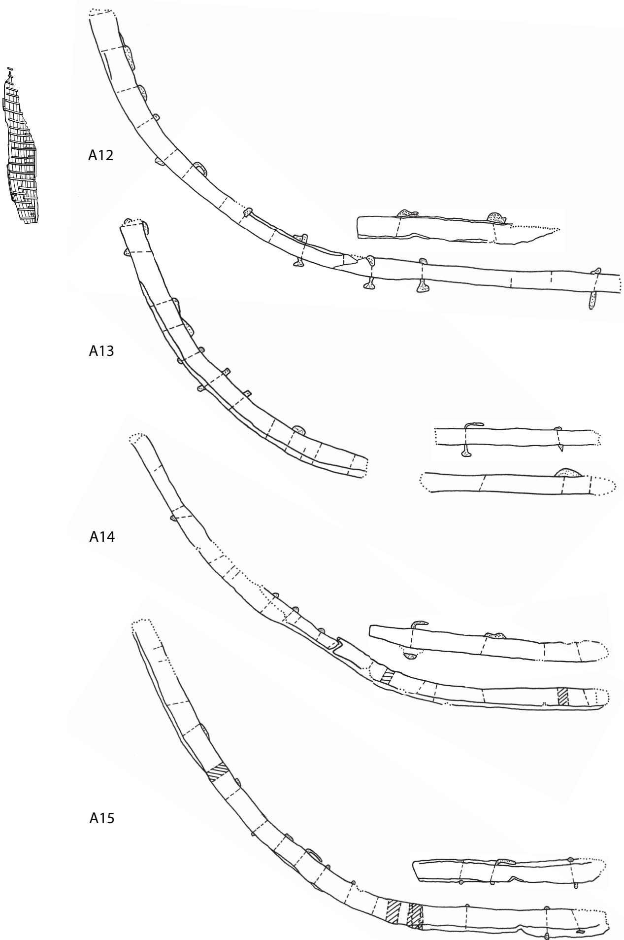
Abb. 56a. – Wrack 2. Spanten A 12* bis A 15*. – M. 1:10.
