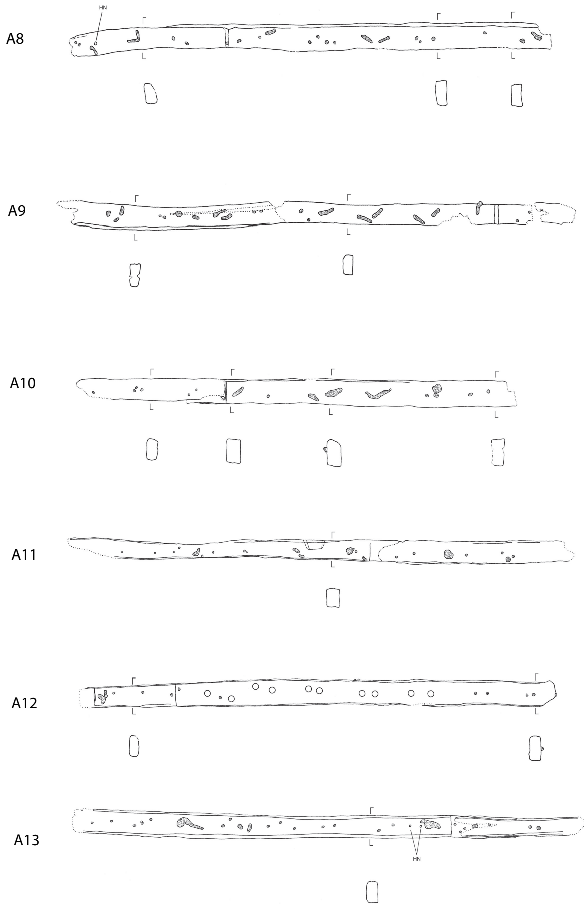
Abb. 61b. – Wrack 3. Spanten A 8 bis A 13. – M. 1:20.
