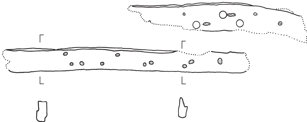
Abb. 57b. – Wrack 2. Spanten A 16* bis A 19*. – M. 1:10.
