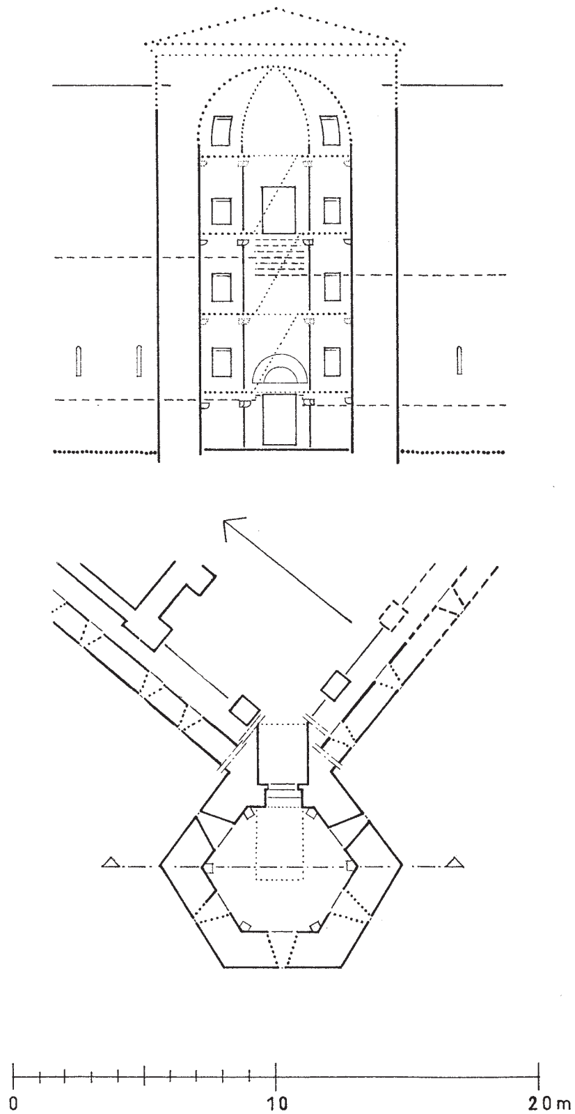
Kastron, Südwestturm, Grundriss und Querschnitt (U. Hess).
