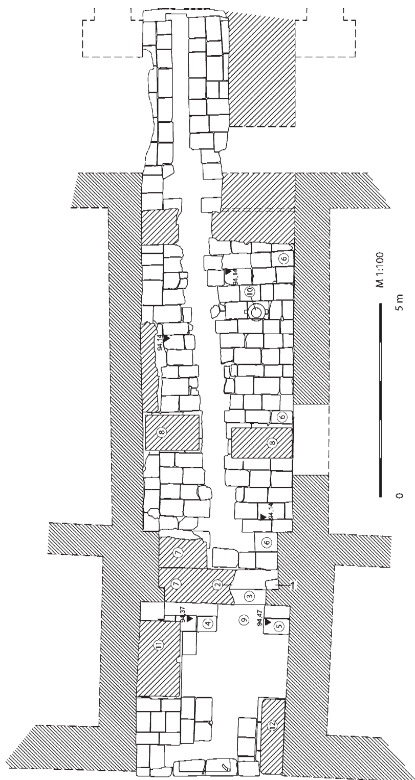
Kastron, Westtoranlage. Grundriss des westlichen Vorraumes und östlichen Vestibüls.
