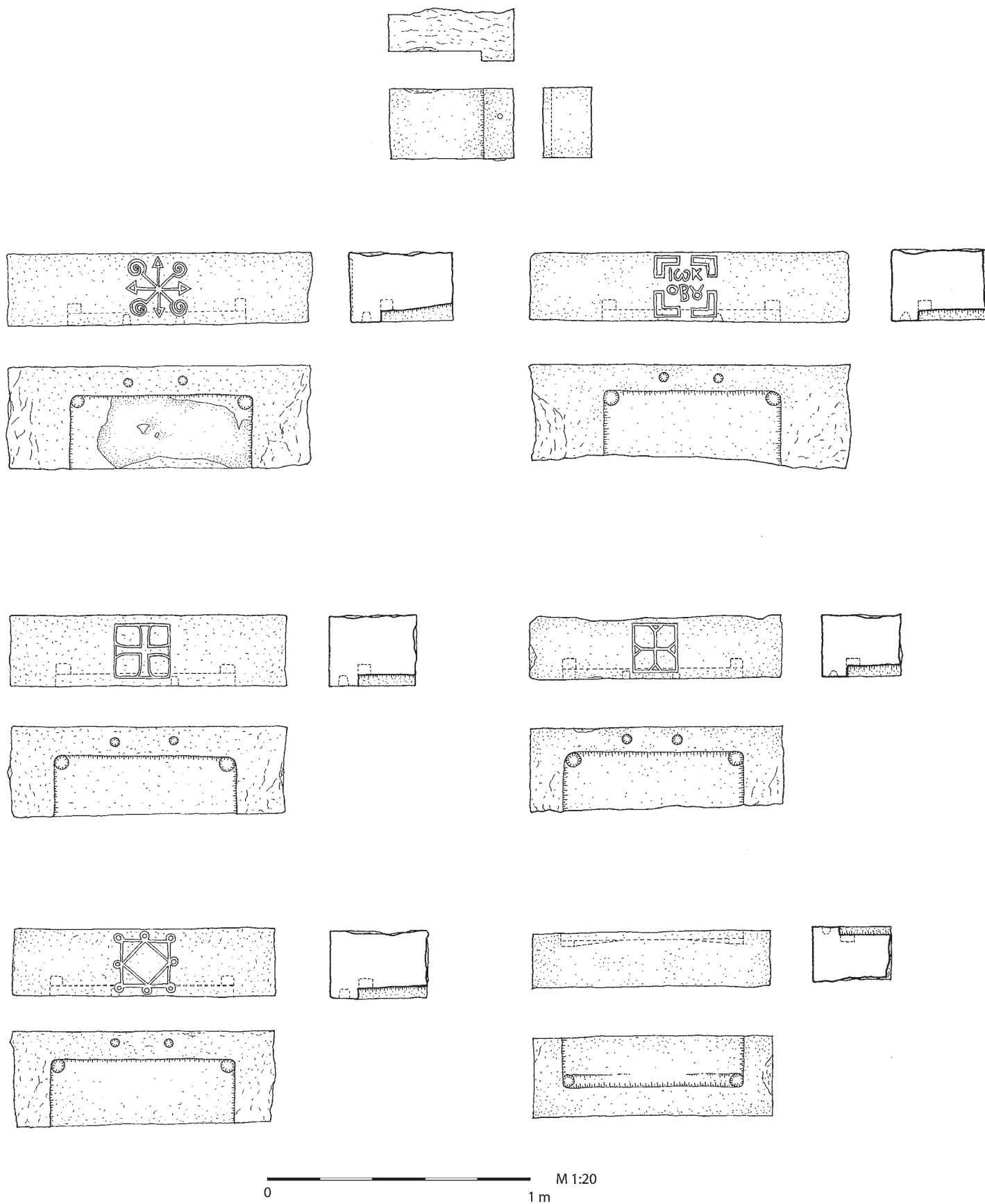
Kastern, Westtrakt. Elemente von sechs Rechteckfenstern aus dem Versturz vor der Südwestmauer.
