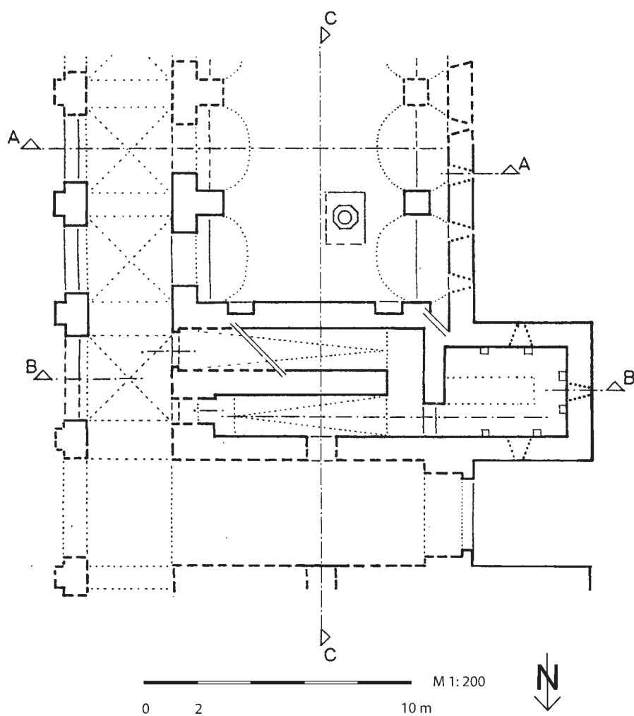
Kastron: 1 Westtrakt. Schnitt durch Portikus, Rampenhaus, Südturm des Westtores (O. Hofmeister). – 2 Grundriss der Rekonstruktionsvorschläge des Westtraktes.
