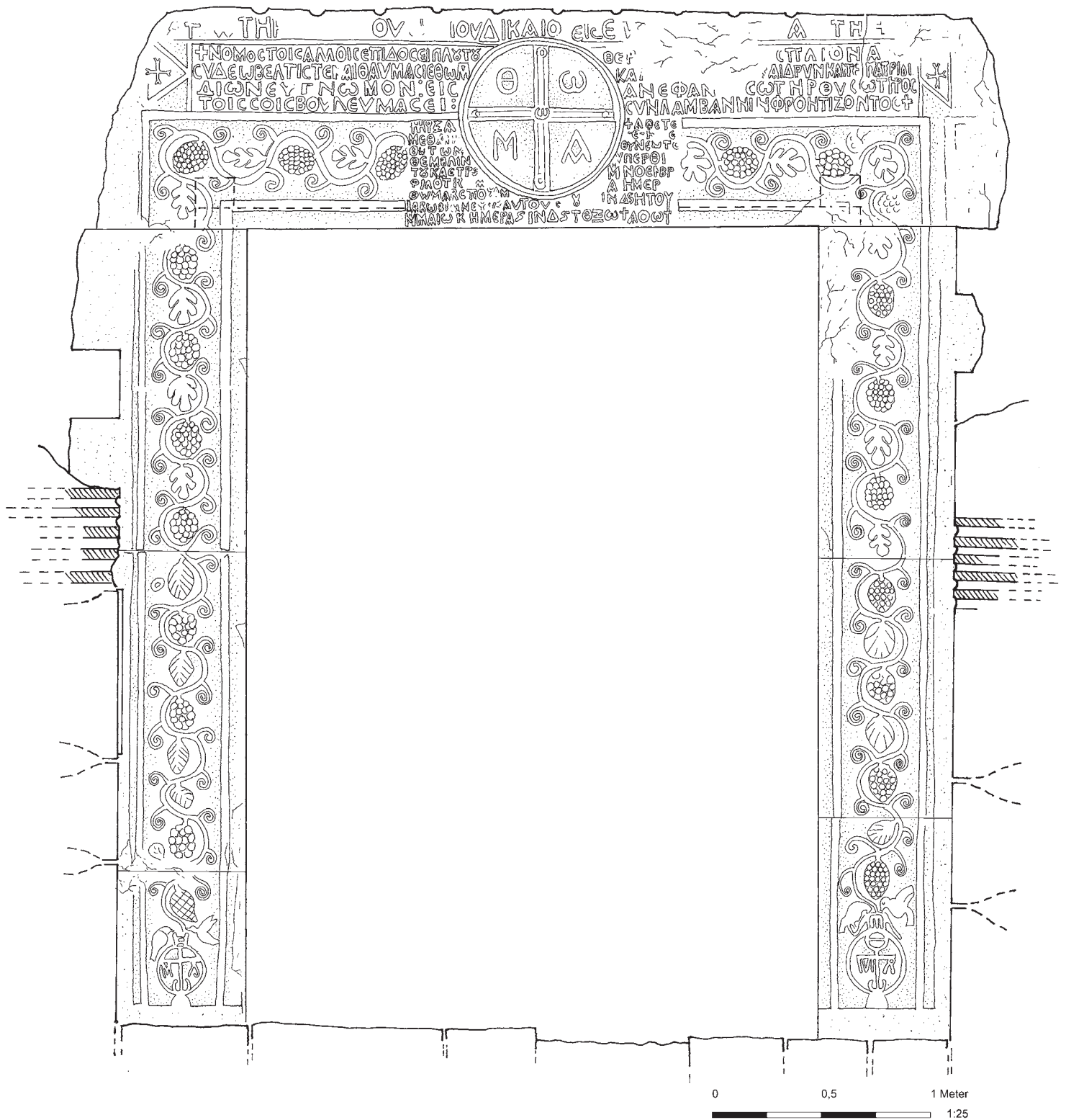
Kastron, Aufnahme der Frontseite des Westtores. – M. 1:25.
