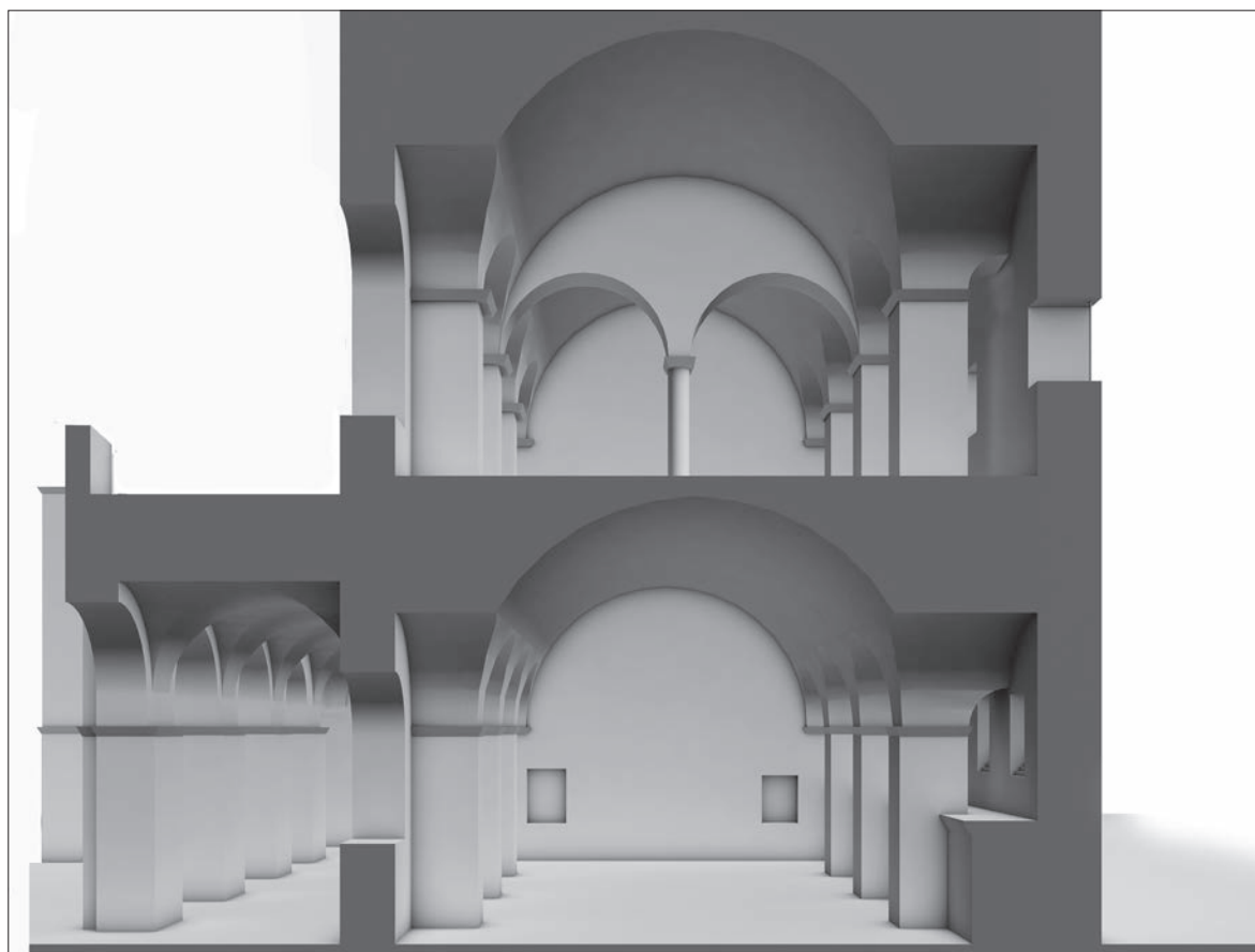
Querschnitt durch Westhalle und Portikus: 1 Blick nach Süden; 2 Variante mit hypothetisch eingesetztem Querteiler im Obergeschoss. – (O. Hofmeister).
