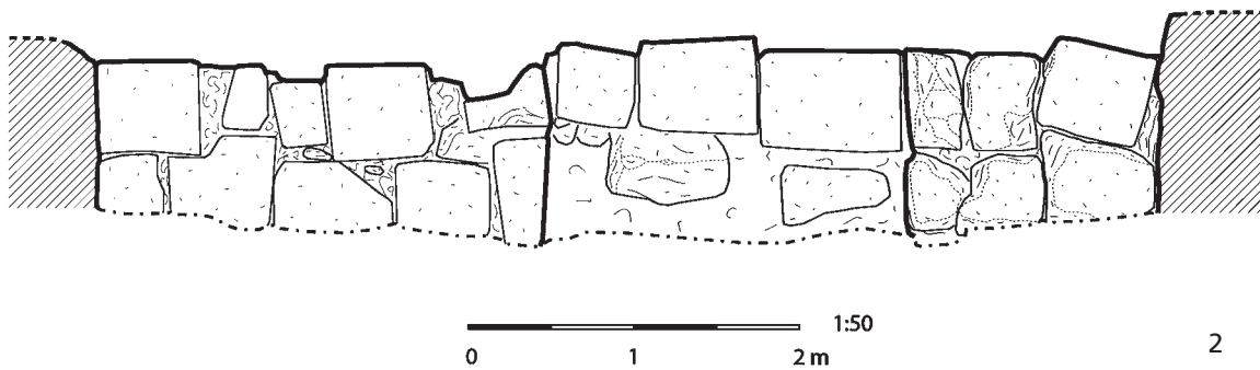
Kastron, Westhalle: 1 Sekundärmauer an der Südseite des Brunnenraums. – 2 Quermauer an der Ostseite des mittleren Kompartiments (5A 2 ).
