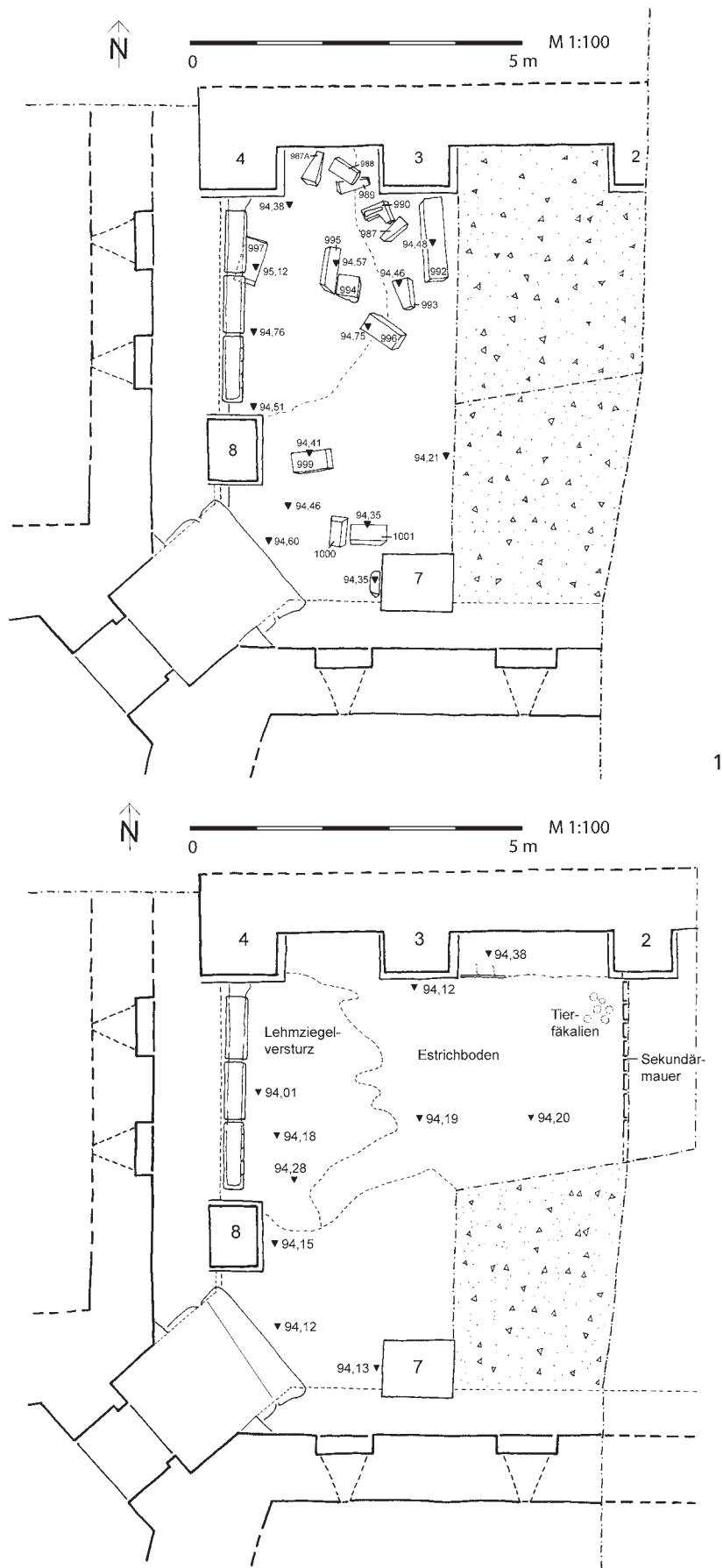
Kastron, Südhalle: 1 Plan der Sondage 8,1. – 2 Plan der Sondage 8,2.
