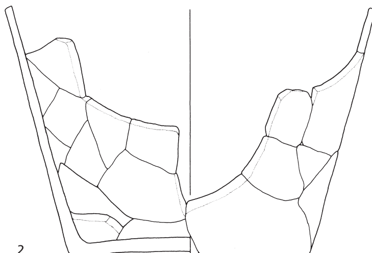
Kleinklein, Kröllkogel: Tonsitulen mit flacher Schulter. – (Zeichnungen M. Windholz-Konrad). – M. 1:3 u. 1:6.
