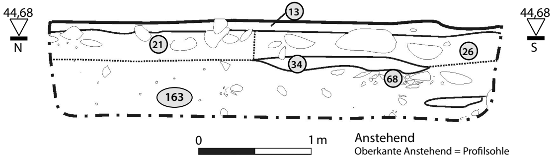
Plan 13: Laubach-Freienseen, Wüstung Baumkirchen, Kirche. N-S-Profil in Fläche 10 (Plan: Ch. Röder).
