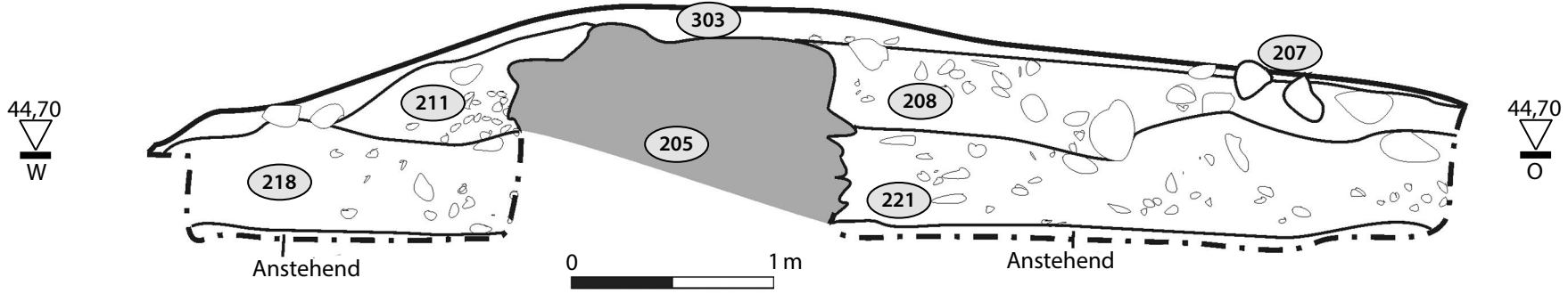
Plan 17: Laubach-Freienseen, Wüstung Baumkirchen, Kirche. W-O-Profil in Fläche 20 (Plan: Ch. Röder).
