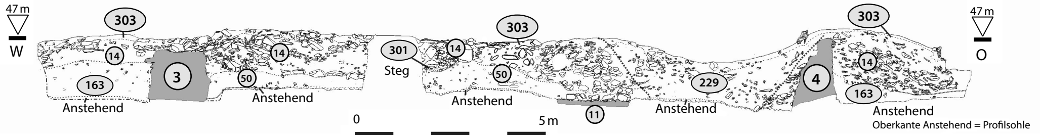
Plan 9: Laubach-Freienseen, Wüstung Baumkirchen, Kirche. W-O-Profil durch den Kirchenbau (Plan: Ch. Röder).
