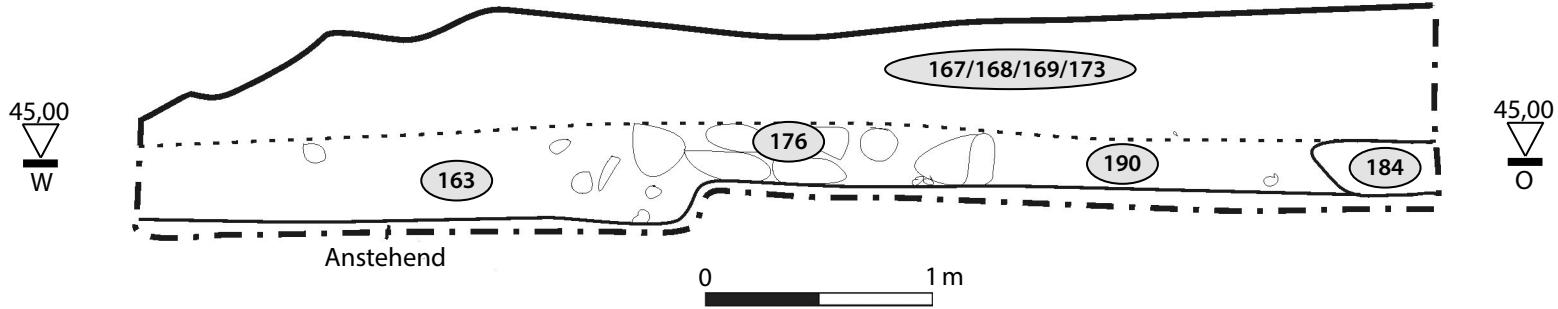
Plan 15: Laubach-Freienseen, Wüstung Baumkirchen, Kirche. W-O-Profil in Fläche 17 (Plan: Ch. Röder).
