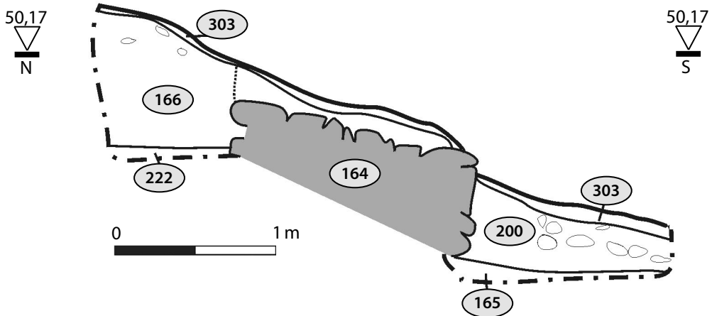
Plan 14: Laubach-Freienseen, Wüstung Baumkirchen, Ausschnitt N-S-Profil in Fläche 16 (Plan: Ch. Röder).
