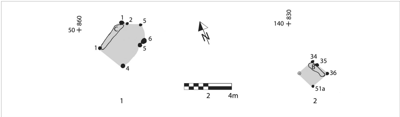
Abb. 17. Pfostenbauten mit Langgruben: (1) in Fläche E87; (2) in Fläche N84, NW-Pfosten ergänzt. Ausschnitte Gesamtplan (Grafik: O. Schlegel).
