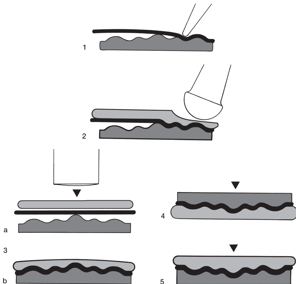
Abb. 59 Herstellung von Pressblechen. – Dunkles Raster: Bronzmodell; helles Raster: Bleiplatte; schwarz: Blech. – 1 Das Blech wird mit einem Metallstift in die Vertiefungen des Pressmodells gepresst. – 2 Das Blech wird durch Hammerschläge auf die Bleiplatte in die Vertiefungen des Pressmodells gepresst. – 3a-b Das Blech wird durch einen einzigen Schlag auf die Bleiplatte in die Vertiefungen des Pressmodells gepresst. – 4 Pressblech zwischen Model und Bleiplatte als Schlagunterlage. – 5 Pressblech zwischen Bleiplatte und Pressmodel mit Negativform. – (Nach Armbruster 2002a, 158 Abb. 34).
