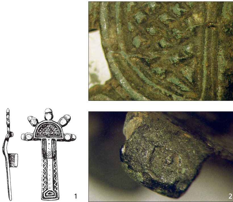
Abb. 39 Halbfertige, bronzene Bügelfibel (1) aus Giberville (dép. Calvados/F) (2 Detail). – (Nach Hincker/Saint Jores/Savary 2005, 54 Abb. 5-7). – 1 M. 1:2; 2 o. M.
