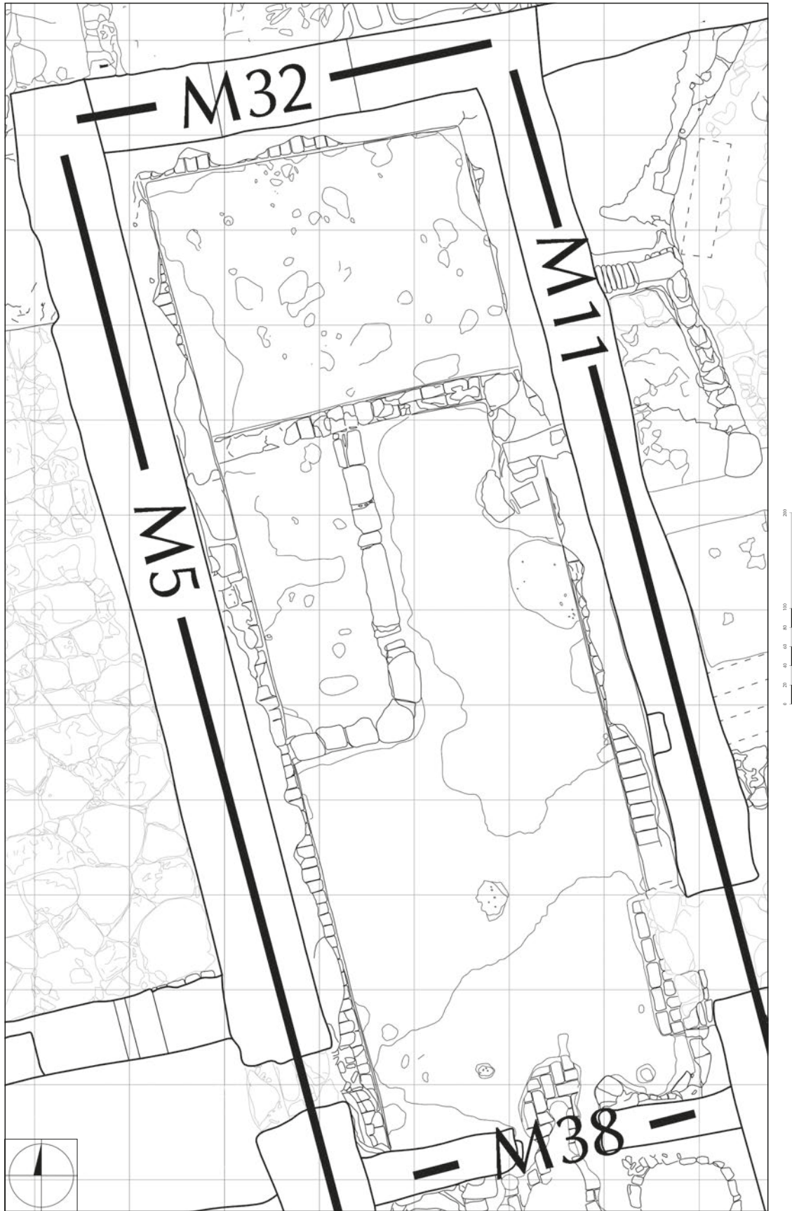
OT_83. Grundrisszeichnung. – (Plan K. Czarnitzki/S. Olschok).
