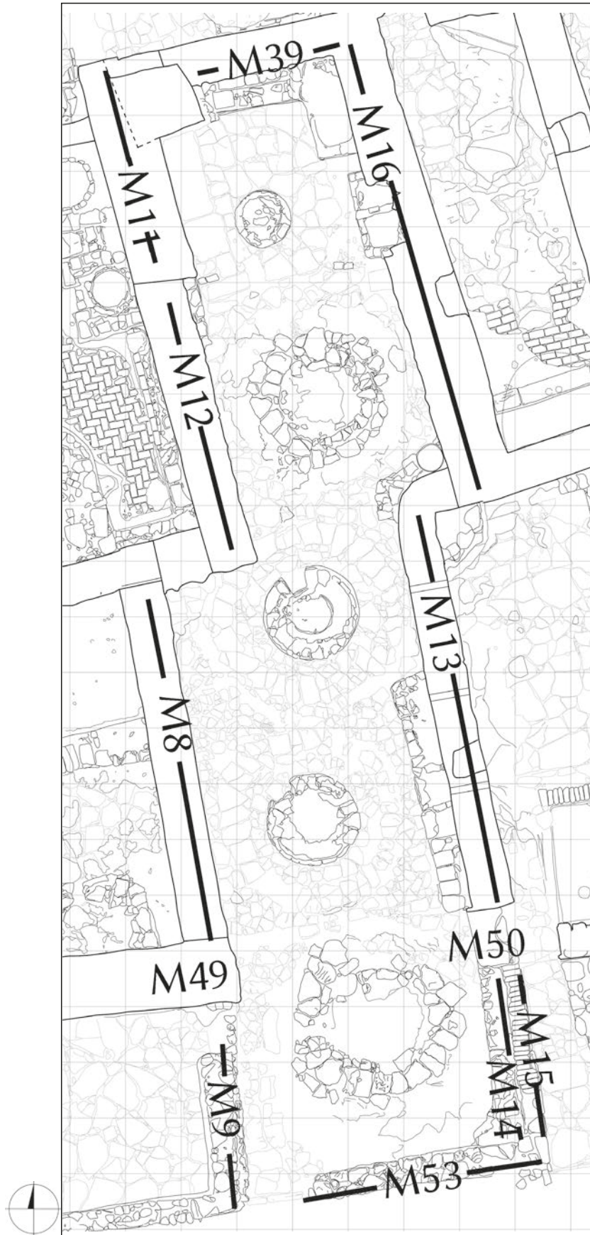
OT_74. Grundrisszeichnung. – (Plan K. Czarnitzki/S. Olschok).
