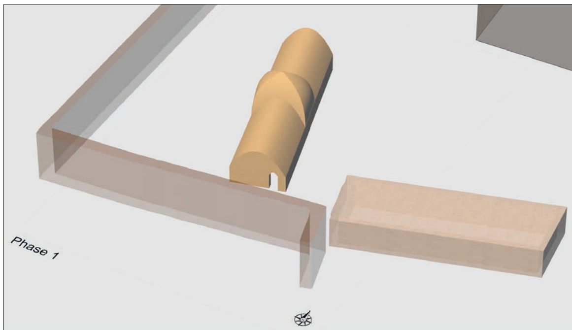
Phase 1 – Rekonstruktionsvorschlag. a Grundriss. – b 3D-Modell. – c Oratorien in Bawit. – (a-b Plan/Modell K. Czarnitzki/S. Olschok; c nach Grossmann, Christliche Architektur Abb. 143).
