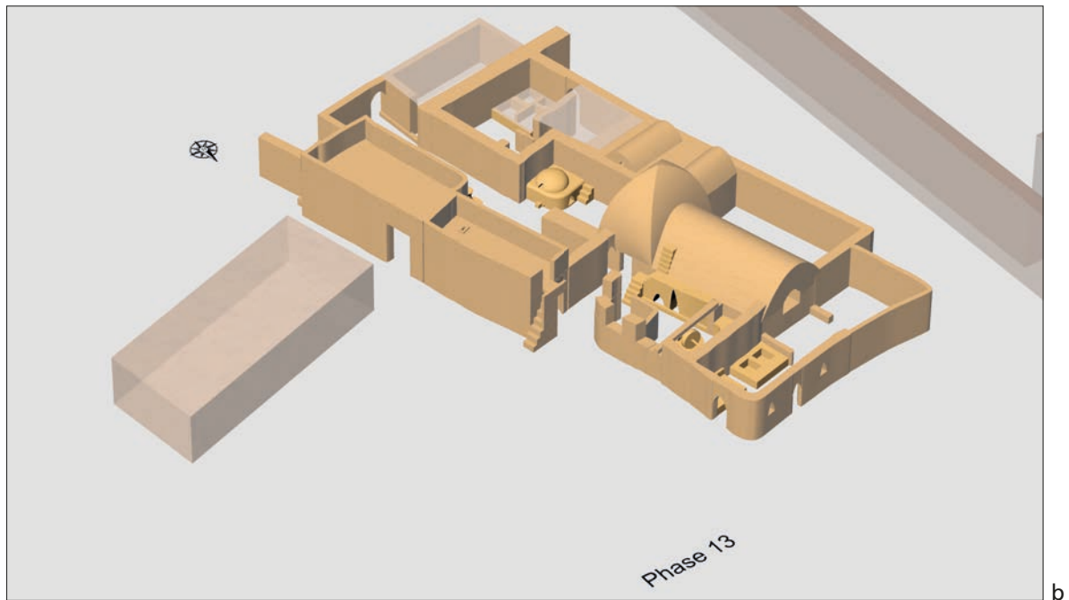
Phase 13 – Rekonstruktionsvorschlag a Grundriss. – b 3D-Modell. – (Plan/Modell K. Czarnitzki/S. Olschok).
