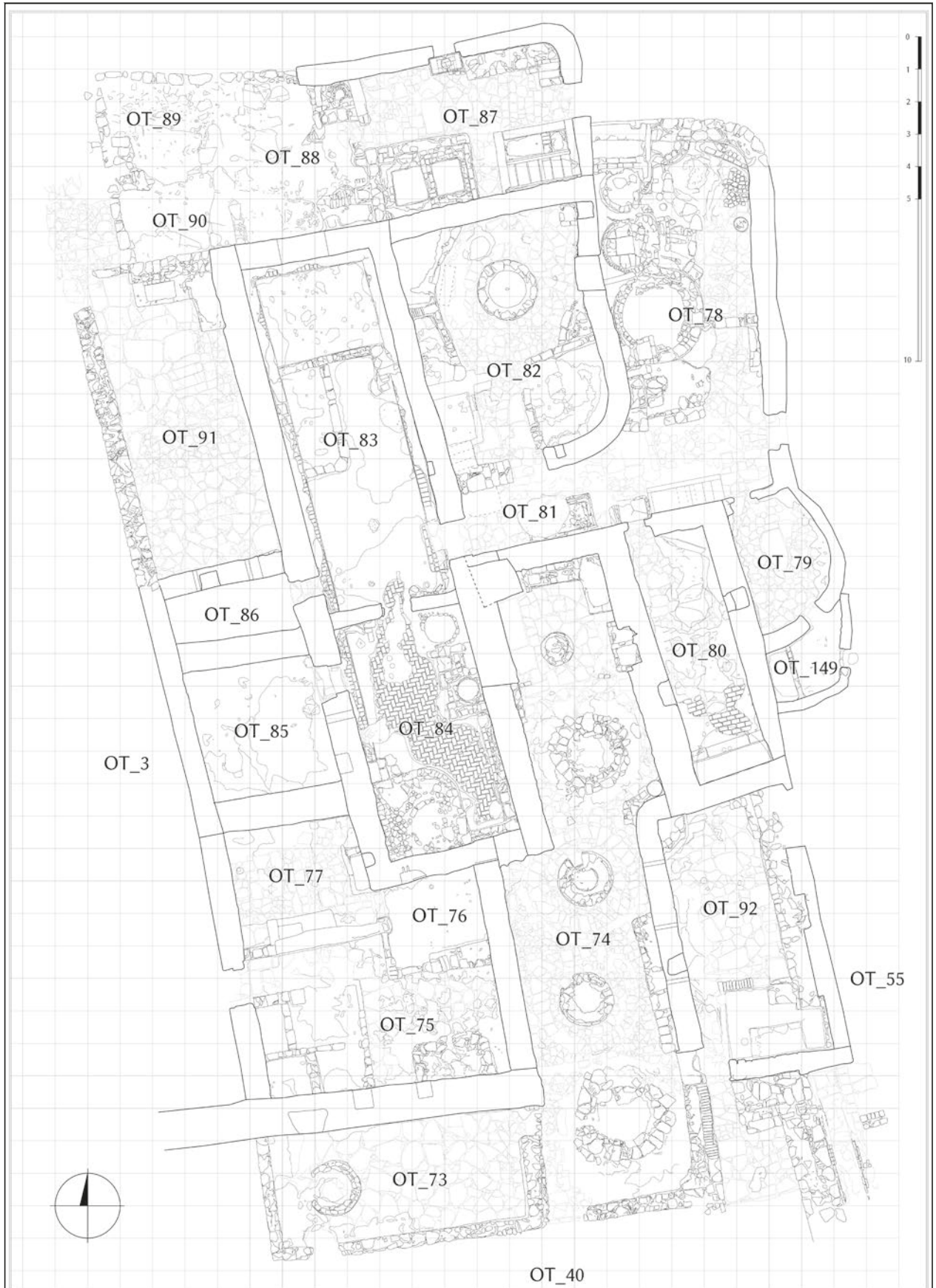
Grundrisszeichnung des Baukomplexes mit Raumnummern.– (Plan K. Czarnitzki/S. Olschok).
