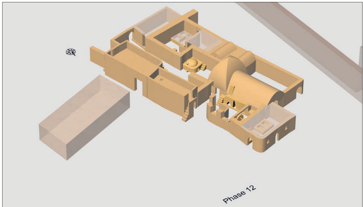
Phase 12 – Rekonstruktionsvorschlag a Grundriss. – b 3D-Modell. – (Plan/Modell K. Czarnitzki/S. Olschok).
