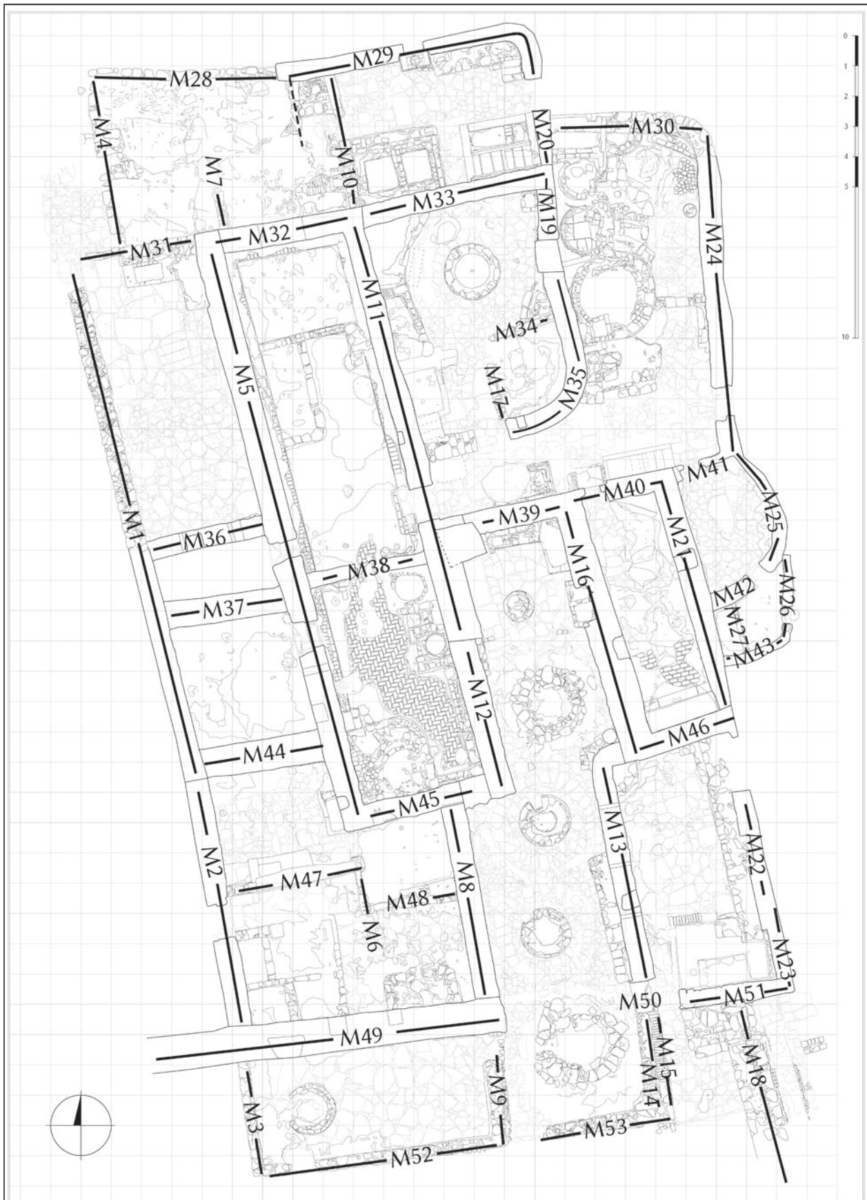
Grundrisszeichnung des Baukomplexes mit Mauernummern. – (Plan K. Czarnitzki/S. Olschok)
