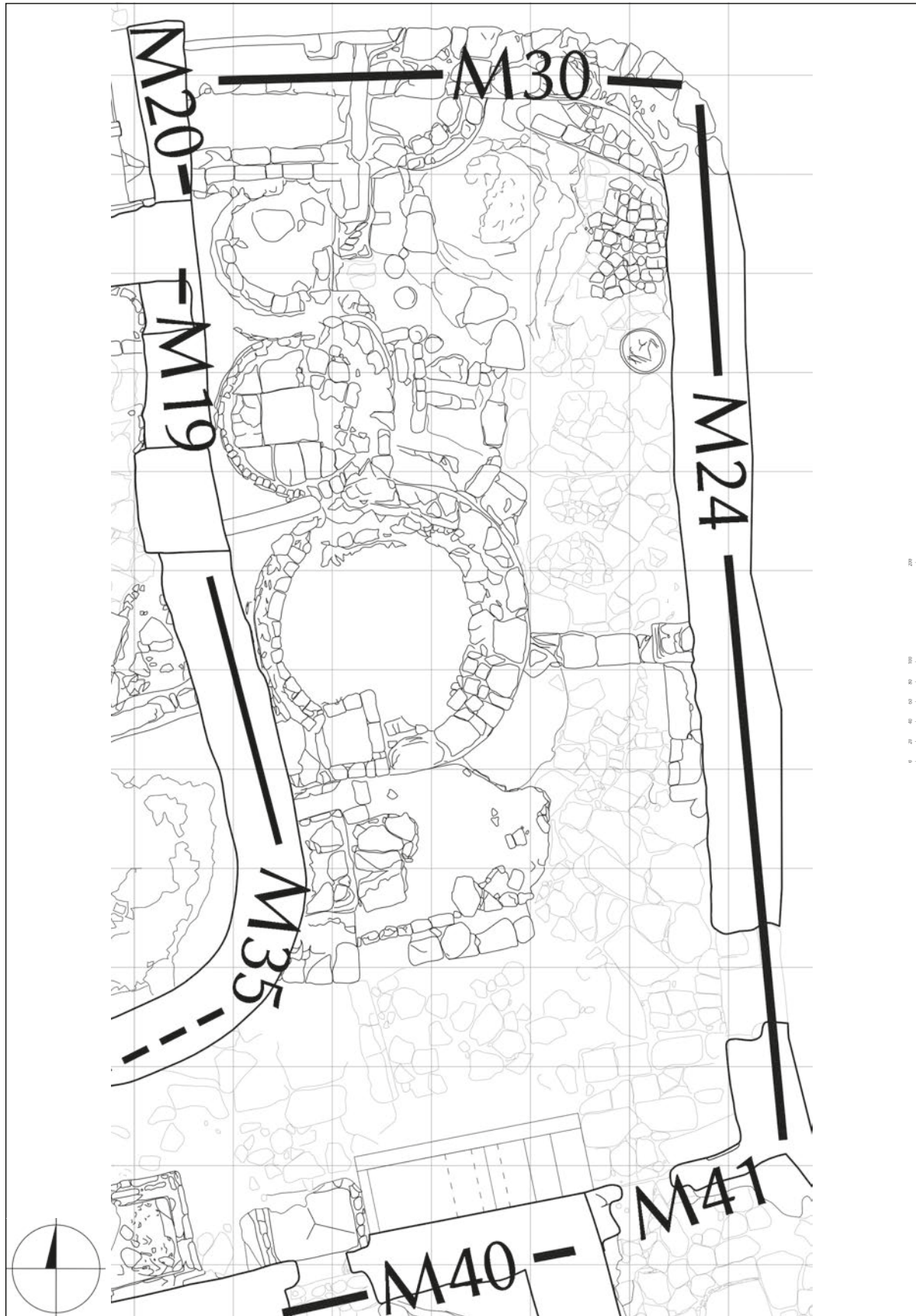
OT_78. Grundrisszeichnung. – (Plan K. Czarnitzki/S. Olschok).
