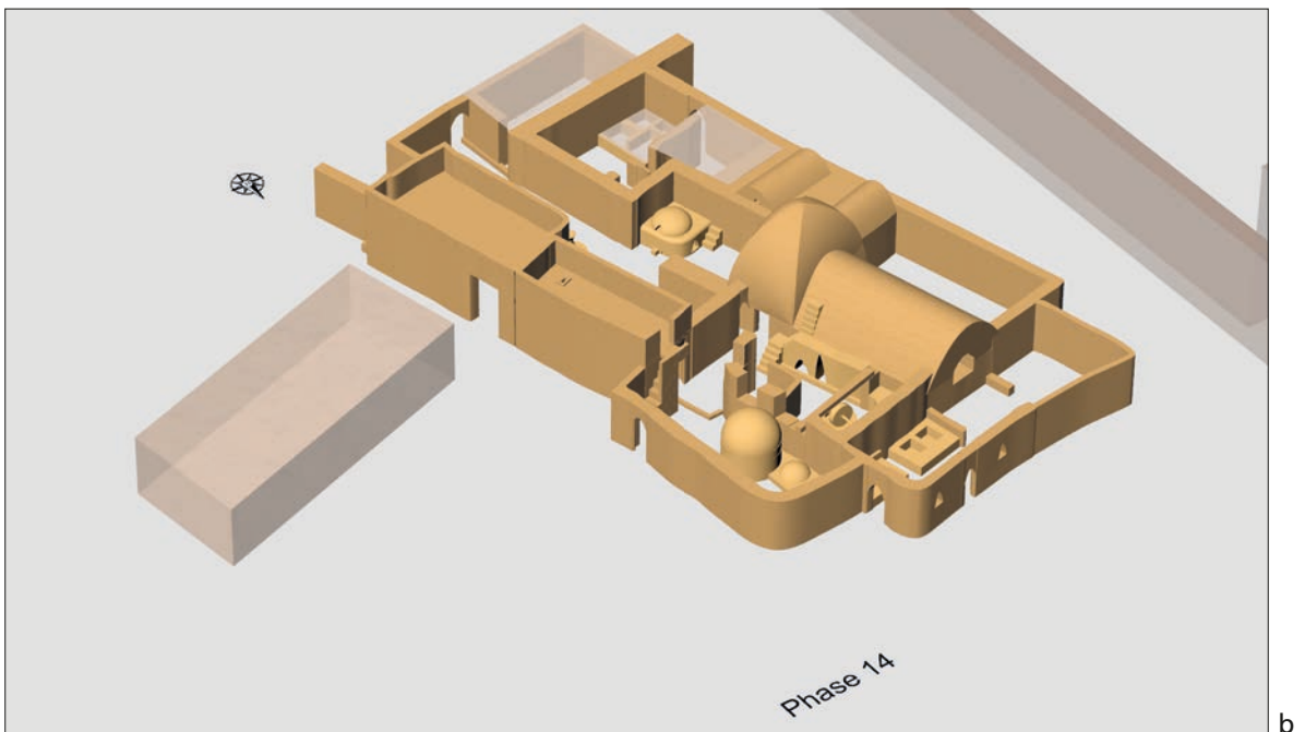
Phase 14 – Rekonstruktionsvorschlag a Grundriss. – b 3D-Modell. – (Plan/Modell K. Czarnitzki/S. Olschok).
