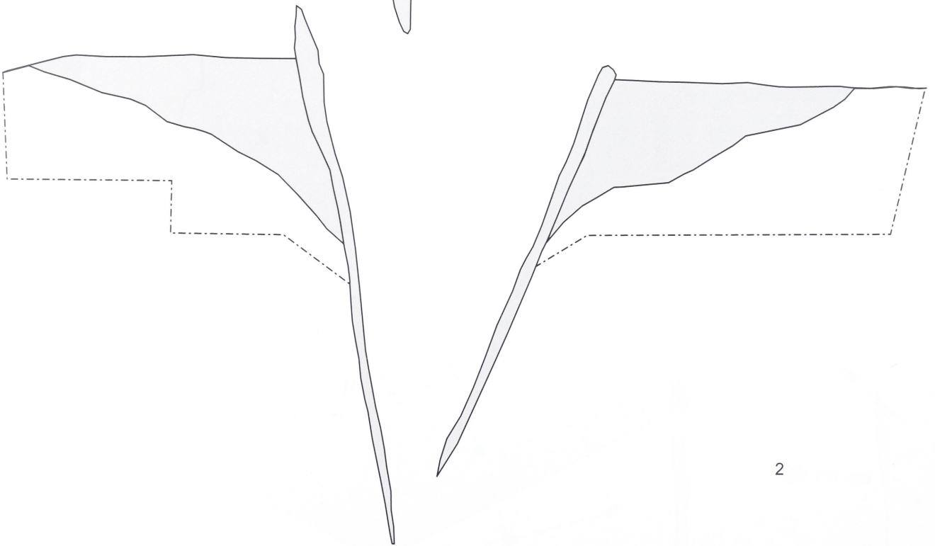
Bergkamen-Oberaden. 1.Bef. 95A/1979, Seitenansicht der Holzverschalung, Blick von Süd; 2.Bef. 95A, Profilschnitt, Blick von Süd. - M. 1:100.
