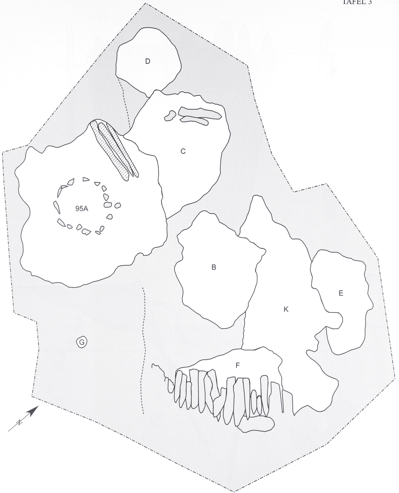
Bergkamen-Oberaden. Bef. 95/1979, Detailplanum (gestrichelte Linie = Unnaer Spannung). - M. 1:50.
