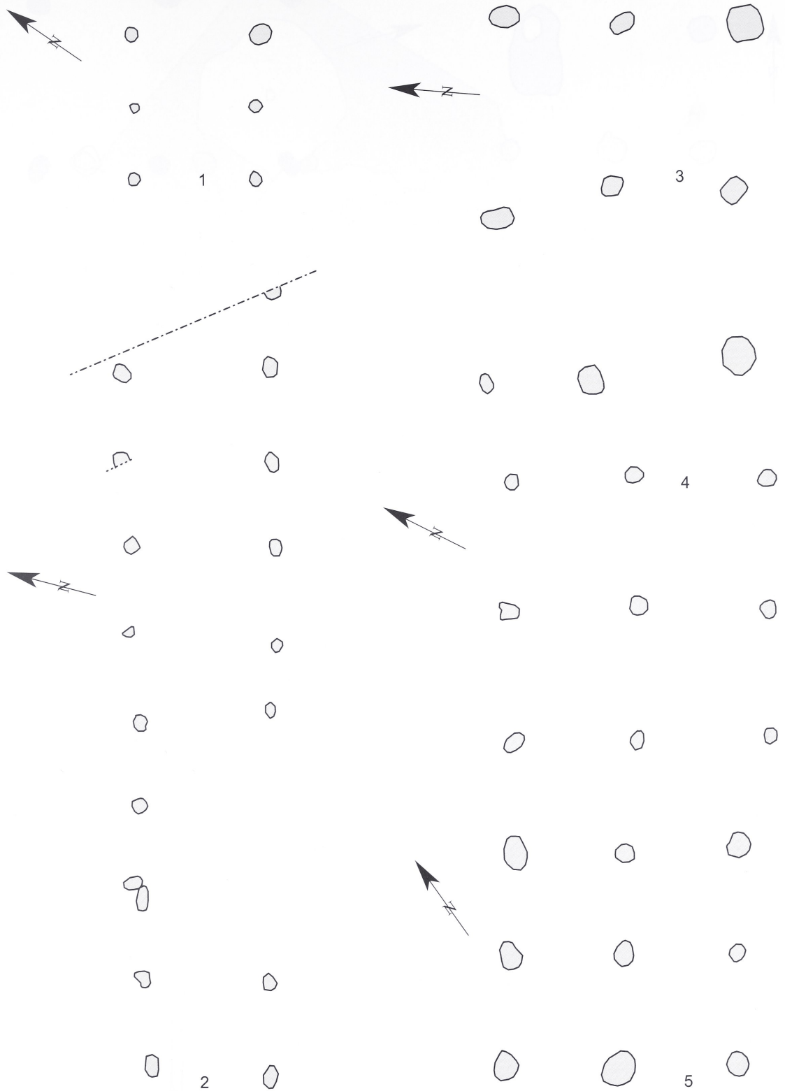
Bergkamen-Oberaden. Gebäudegrundrisse 1-5. - M. 1:100.
