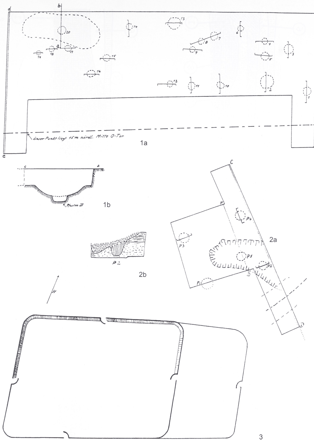
Rüthen-Kneblinghausen. 1a. Arbeitsfeld III O/1938, Planum; 1b. Grube 25 mit Pfosten 20, Profil; 2a. Arbeitsfeld V W/1938, Planum; 2b. Grube 34 mit Pfosten 2, Profil; 3. Verbreitung der "Kulturschicht unter dem Walle"; - 1a, 2a M. 1:100; 1b, 2b M. 1:40.
