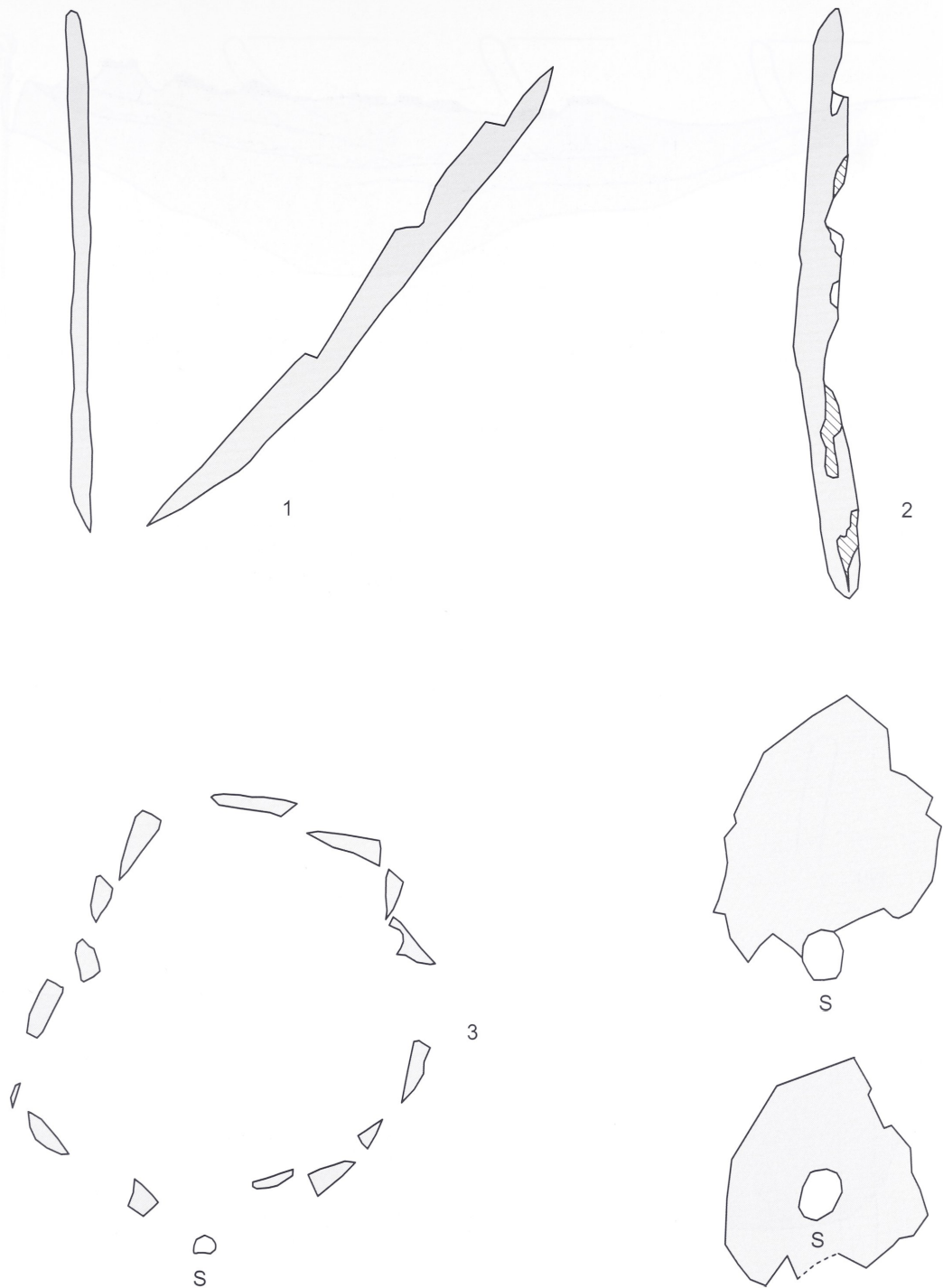
Bergkamen-Oberaden. 1. Bef. 95A/1979, Position des Steigbaums im Brunnenschacht, Blick von West; 2. Bef. 95A/1979, Steigbaum, stellenweise fehlende Rinde (Schraffur); F3. Bef. 95A/1979, Querschnitt des Brunnenschachtes auf 61,33 m ü. NN (a), 60,43 m ü. NN (b) und 59,93 m ü. NN (c), S = Steigbaum. - M. 1:20.
