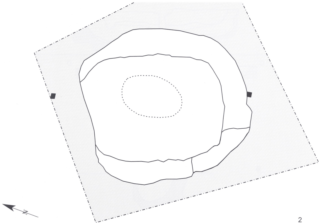
Delbrück-Anreppen (Dkz. 4217,75), 1. Pfostengrundriß; 2. Bef. 1, "Brunnen", Aufsicht 0,15 m unter Hauptplanum. - 1 M. 1:100; 2 M. 1:20.
