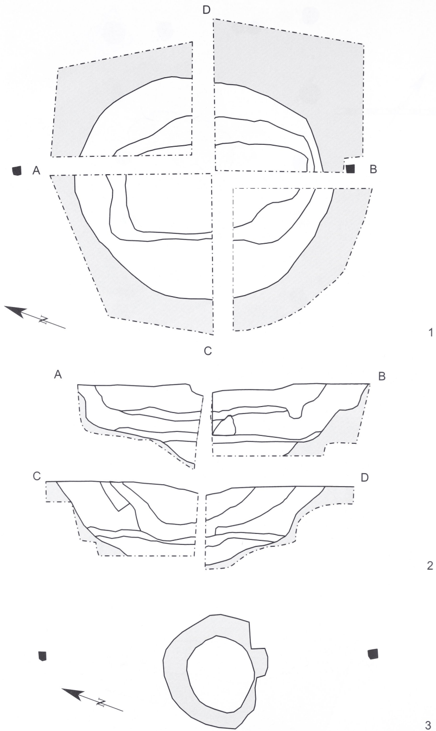
Delbrück-Anreppen (Dkz. 4217,75). 1. Bef. 1, "Brunnen", Aufsicht 0,42 m unter Hauptplanum; 2. Bef. 1, "Brunnen", Profilansichten; 3. Bef. 1, "Brunnen"; Ansicht 1,15 m unter Hauptplanum. - M. 1:20.
