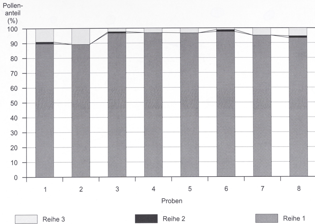
Delbrück-Nordhagen, Pollenprofil.
