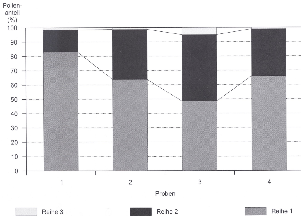
Salzkotten-Mantinghausen, Pollenprofil.
