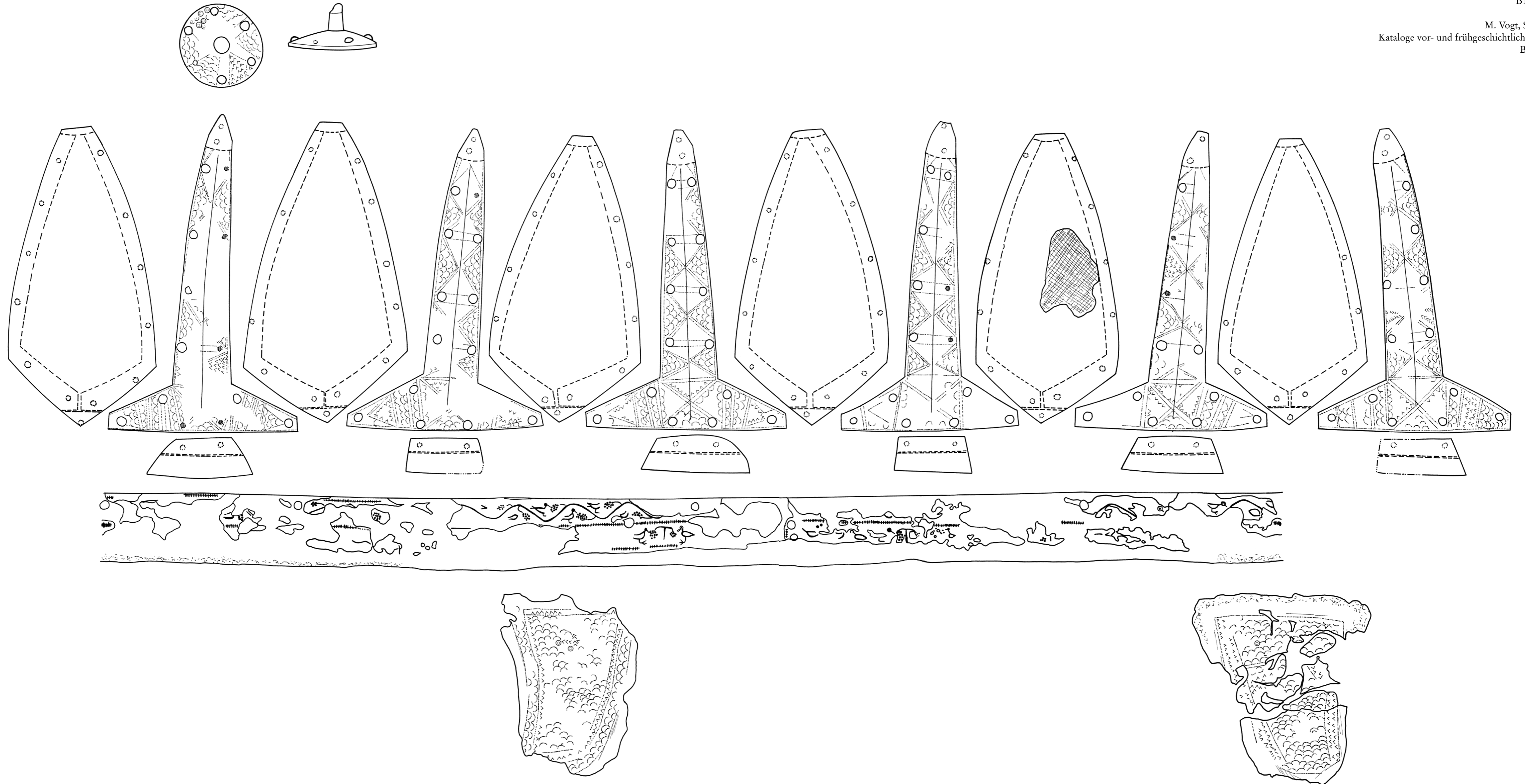
Gültlingen, Abrollung des Helmkörpers M = 2:3
