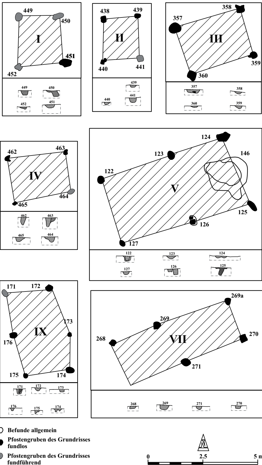
Bauten I, II, III, IV, V, VII, IX der vorrömischen Eisenzeit und der römischen Kaiserzeit. M 1:100.
