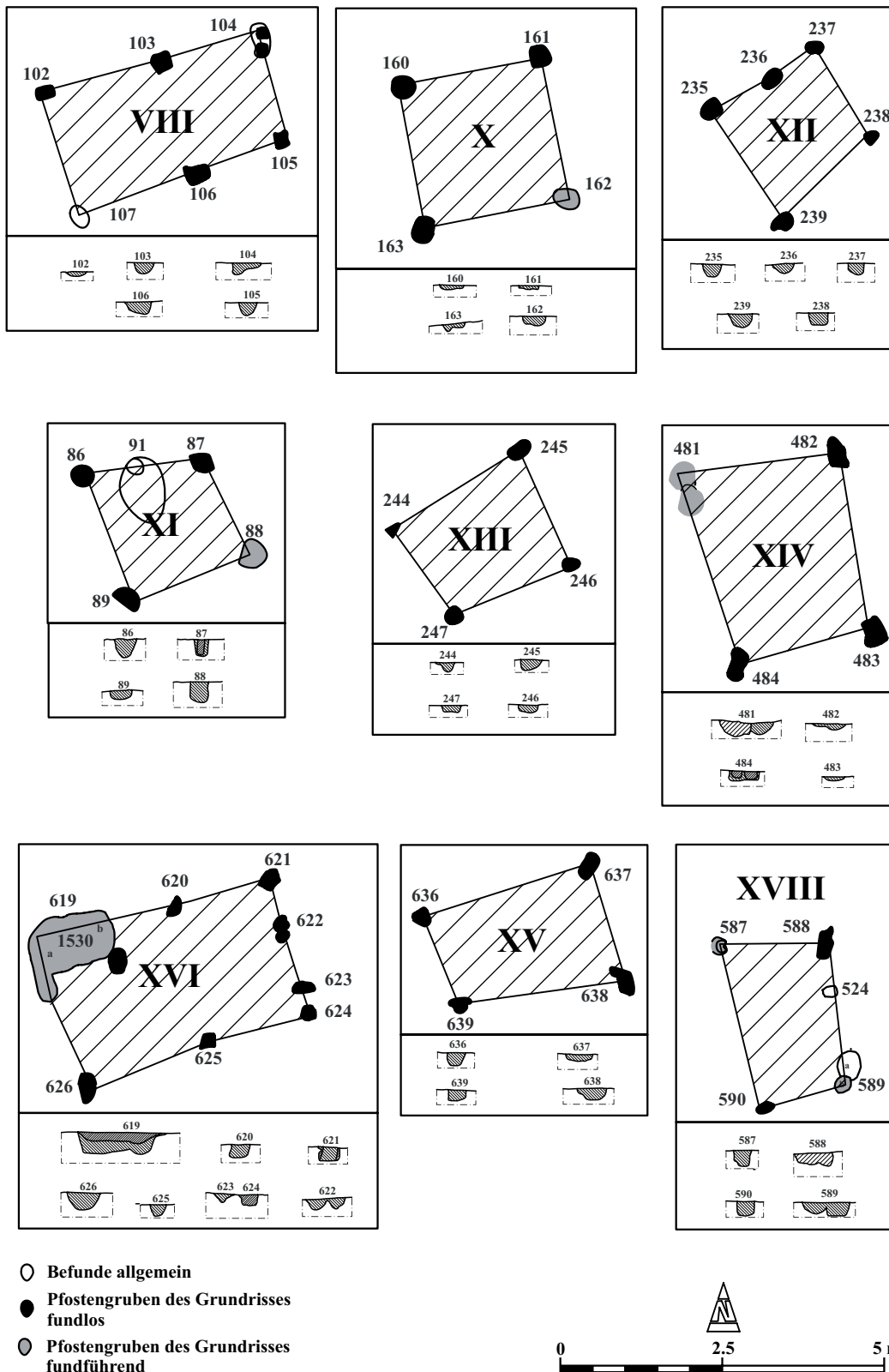
Bauten VIII, X–XVI, XVIII der vorrömischen Eisenzeit und der römischen Kaiserzeit. M 1:100.
