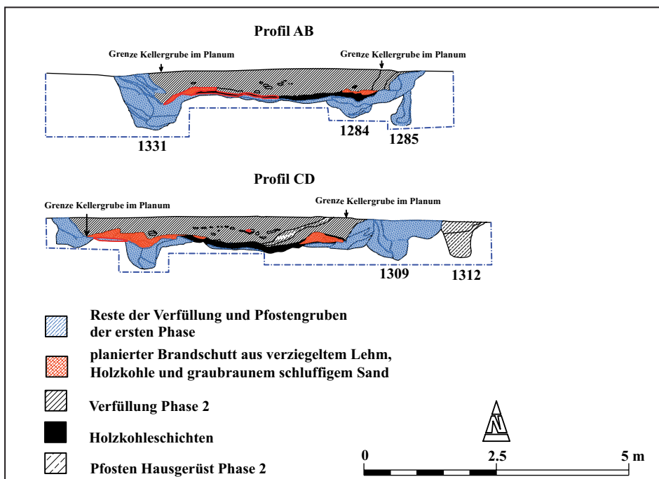
Hochmittelalterlicher Grubenkeller 1283 und Bau 13. M 1:100.
