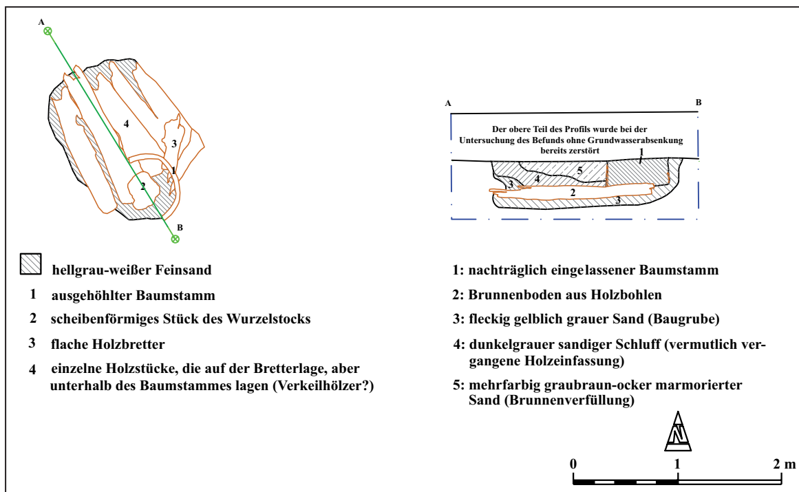
Hochmittelalterlicher Brunnen 1806. M 1:50.
