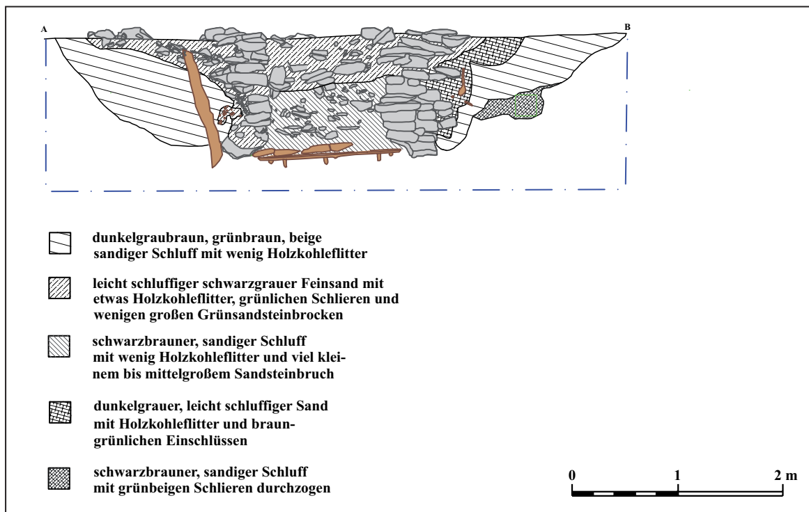
Hochmittelalterlicher Brunnen 1753, Profil. M 1:50.
