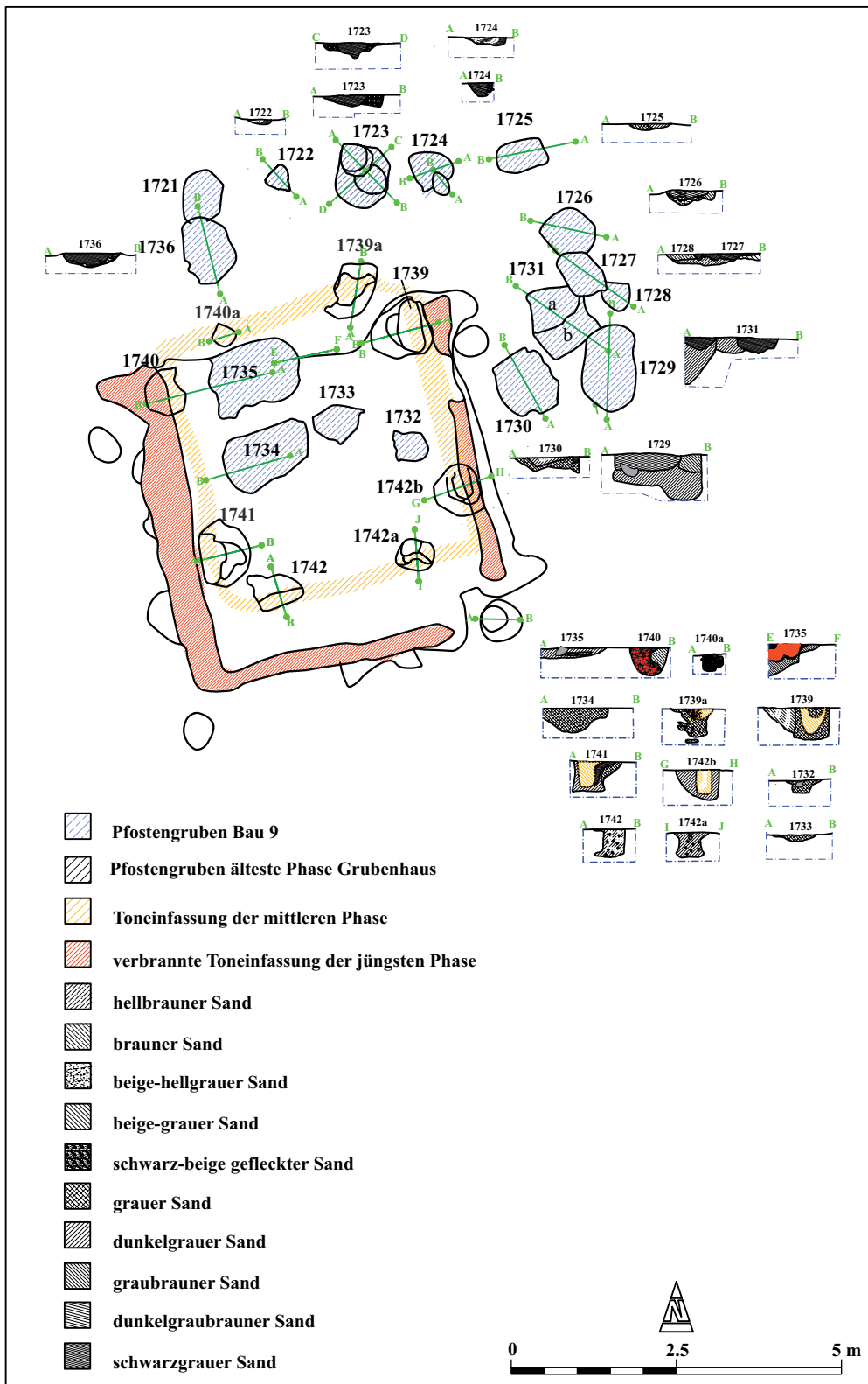
Die Pfostengruben der drei Phasen des hochmittelalterlichen Grubenhauses 1738 und des Kleinbau 9. M 1:100.
