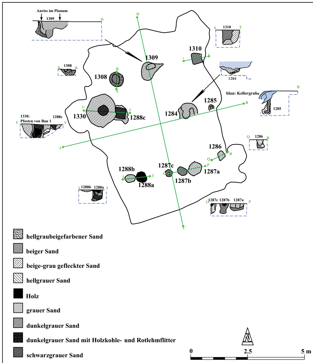
Pfostengruben der älteren Kellerphase des hochmittelalterlichen Kleinbaus 13. M 1:100.
