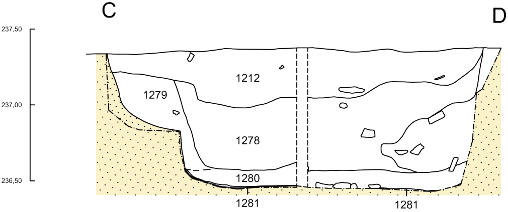
Keller 2 (Schnitt 31/36). Grundriss M 1:50; Profile M 1:25.
