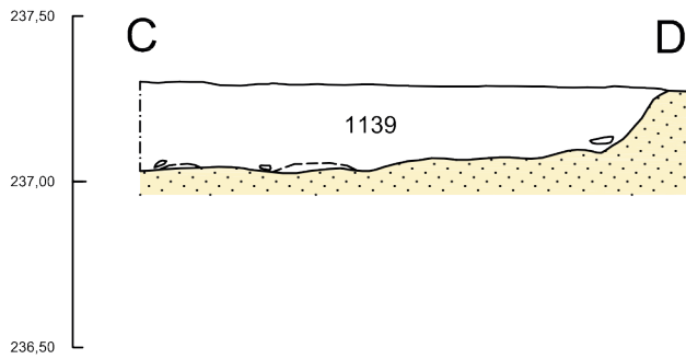
Grubenhaus 12 (Schnitt 23/47). Grundriss M 1:50; Profile M 1:25.
