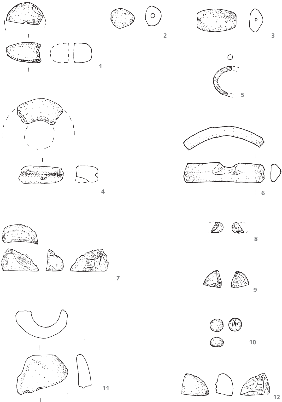
1: Fund-Nr. 463 (Kap. 8.2.6, 1), Bef. 1101; 2: Fund-Nr. 558 (Kap. 8.2.7, 1), Bef. 1736; 3: Fund-Nr. 1525 (Kap. 8.2.7, 2), Bef. 2396; 4: Fund-Nr. 464 (Kap. 8.1.1, Haus C), Bef. 732; 5: Fund-Nr. 150 (Kap. 8.2.5, 1), Bef. 530; 6: Fund-Nr. 707 (Kap. 8.2.5, 6), Bef. 1915; 7: Fund-Nr. 1540 (Kap. 8.2.5, 17), Schnitt 33; 8: Fund-Nr. 461 (Kap. 8.2.5, 5), Bef. 1108; 9: Fund-Nr. 1565 (Kap. 8.2.5, 21), Bef. 1654; 10: ohne Fund-Nr. (Kap. 8.2.5, 27), Bef. 2754; 11–12: ohne Fund-Nr. (Kap. 8.2.5, 30), Schnitt 27. M 1:1.
