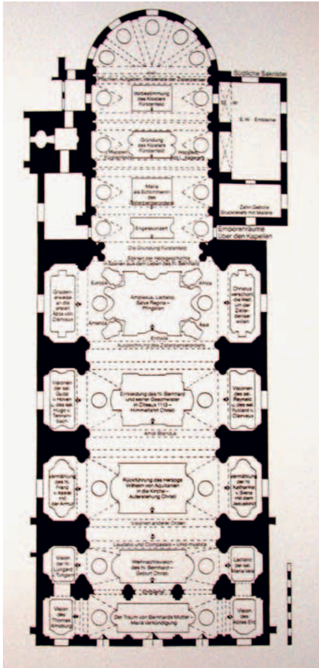
Abb. 5 Fürstenfeld, ehem. Zisterzienserabtei St. Maria Himmelfahrt, Grundriss
