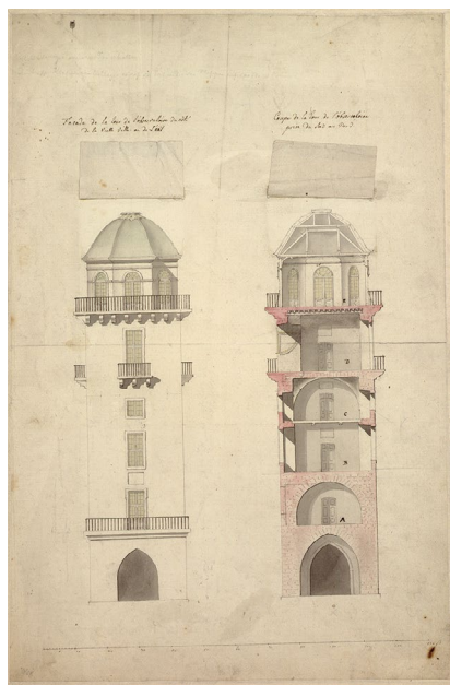
Abb. 65 S.L. du Ry, Entwurf für Zehrenturmumbau 1779, Facade de la tour de l'observatoire du côté de la vieille ville ou de l'est, 1779, (jeweils links auf beiden Blättern unten), Coupe de la tour de l'observatoire prise du Sud au Nord, (jeweils rechts auf beiden Abbildungen unten) mit aufgeklebter Änderung für die Umwandlung der Kuppel in eine Plattform, Quelle: HStAM
