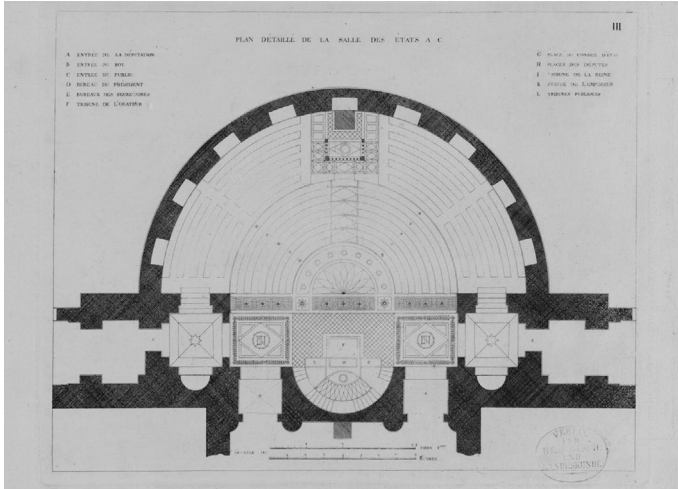
Abb. 117 Auguste-Henri-Victor Grandjean de Montigny, „Plan, Coupe, Élévation et détails [...]”, Cassel 1810, Planche III: Plan détaillé de la Salle des États A C, Quelle: MHK, Graphische Slg.
