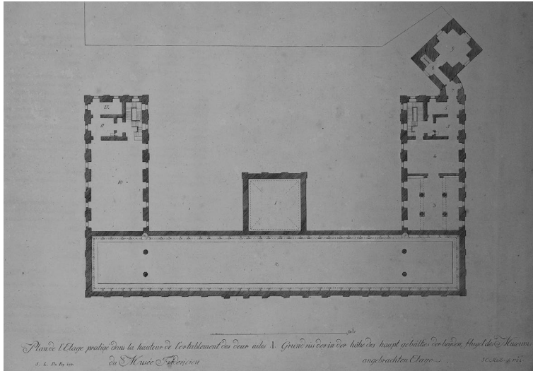
Abb. 23 J.G. Fünck/S.L. du Ry/J.C. Müller/G.W. Weise, Stichwerk Plans et vüe perspective [...], 1784, Plan de l'Etage pratique dans la hauteur de l'entablement des deux ailes, Quelle: WLB
