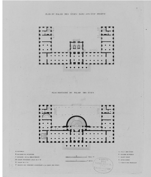
Abb. 115 Auguste-Henri-Victor Grandjean de Montigny, „Plan, Coupe, Élévation et détails de la restauration et détails de la restauration du Palais des États et de sa nouvelle salle à Cassel“, Cassel 1810, Planche I: Plan du Palais des Etats dans son état primitif/Plan restauré du Palais des Etats, Grundriss des Ständepalasts vor und nach dem Umbau 1810, Quelle: MHK, Graphische Slg.
